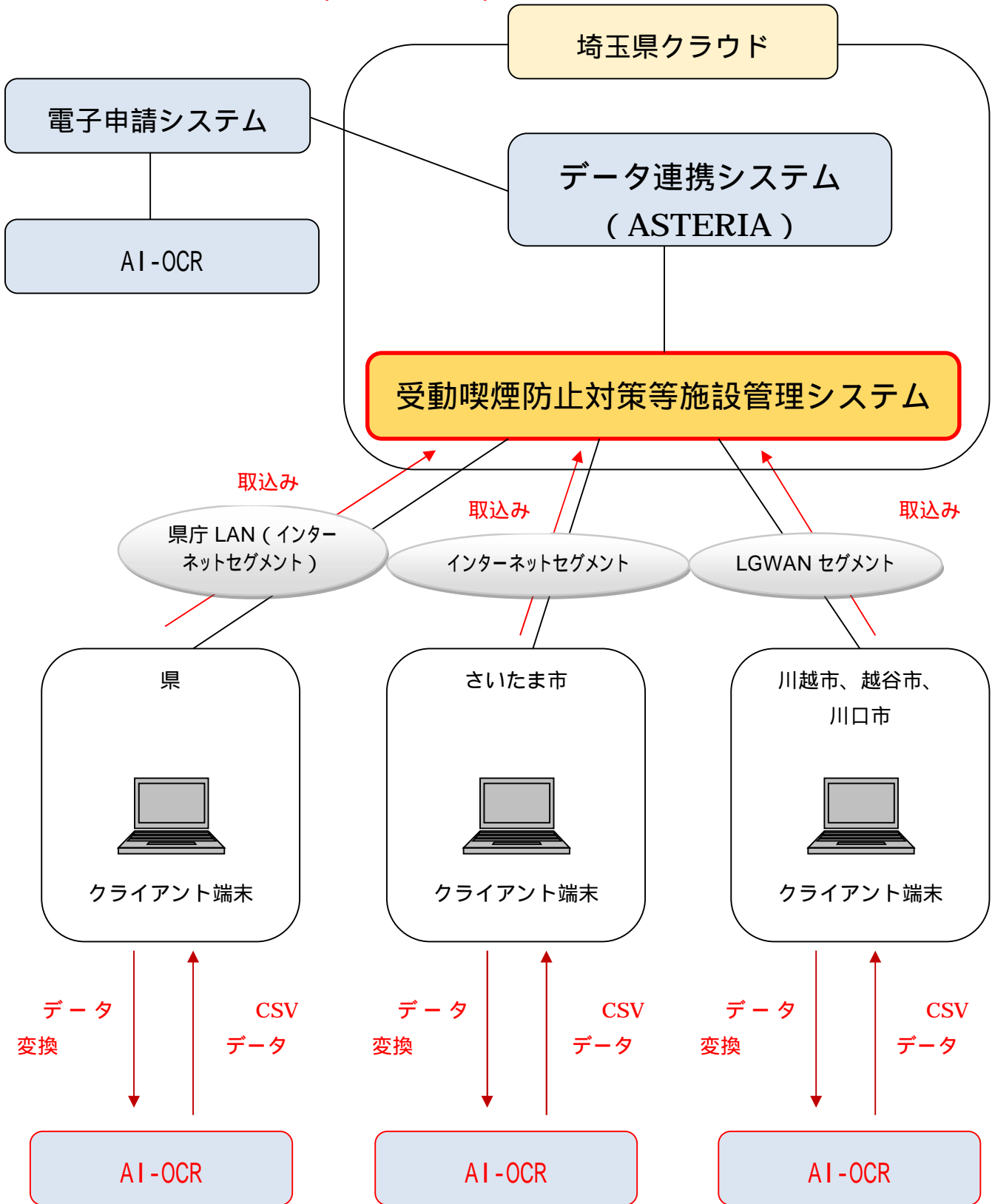
機器ネットワーク構成図 (赤字部分加筆)
