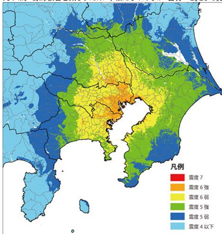
震度分布（都心南部直下地震）
