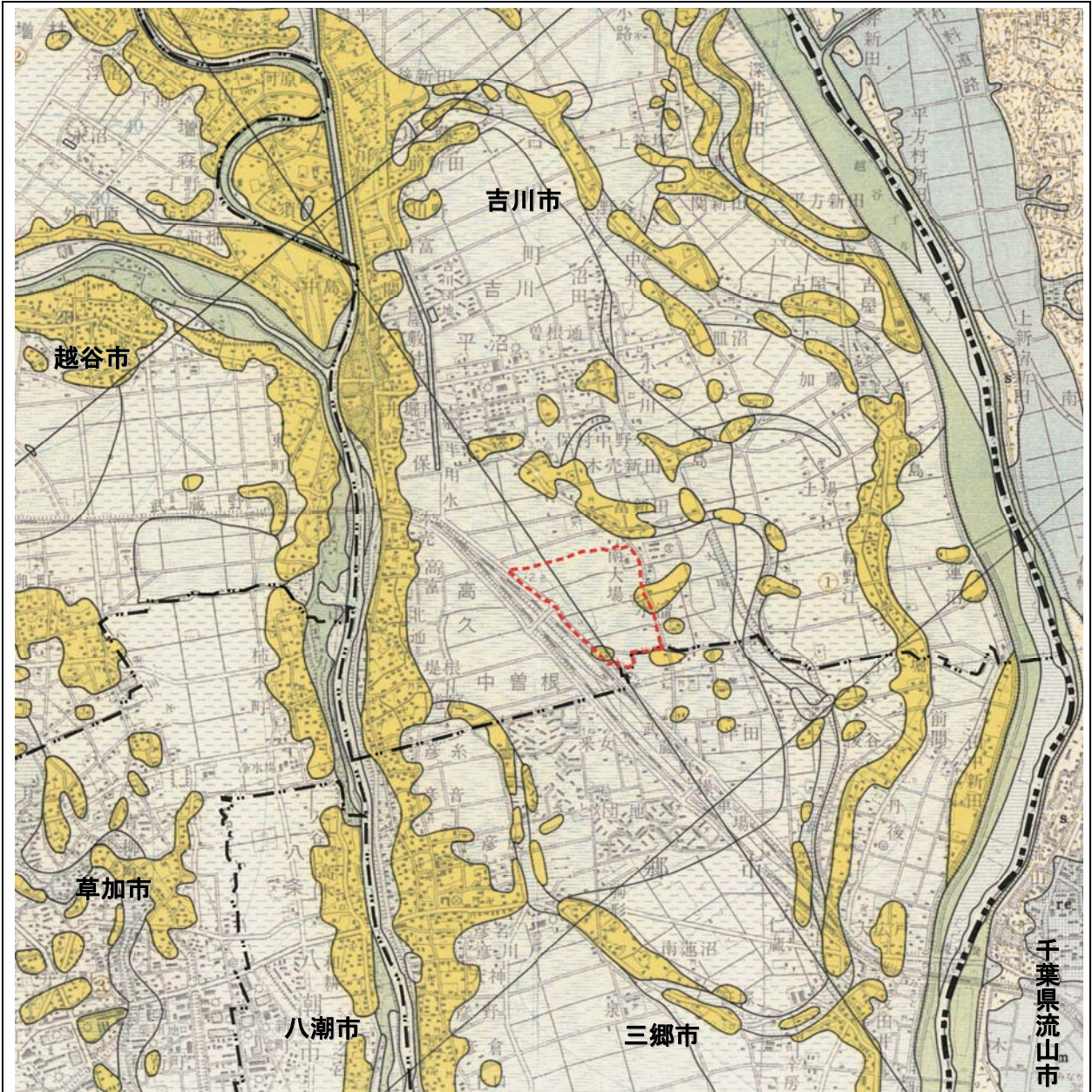
図 3-2-7 表層地質図
