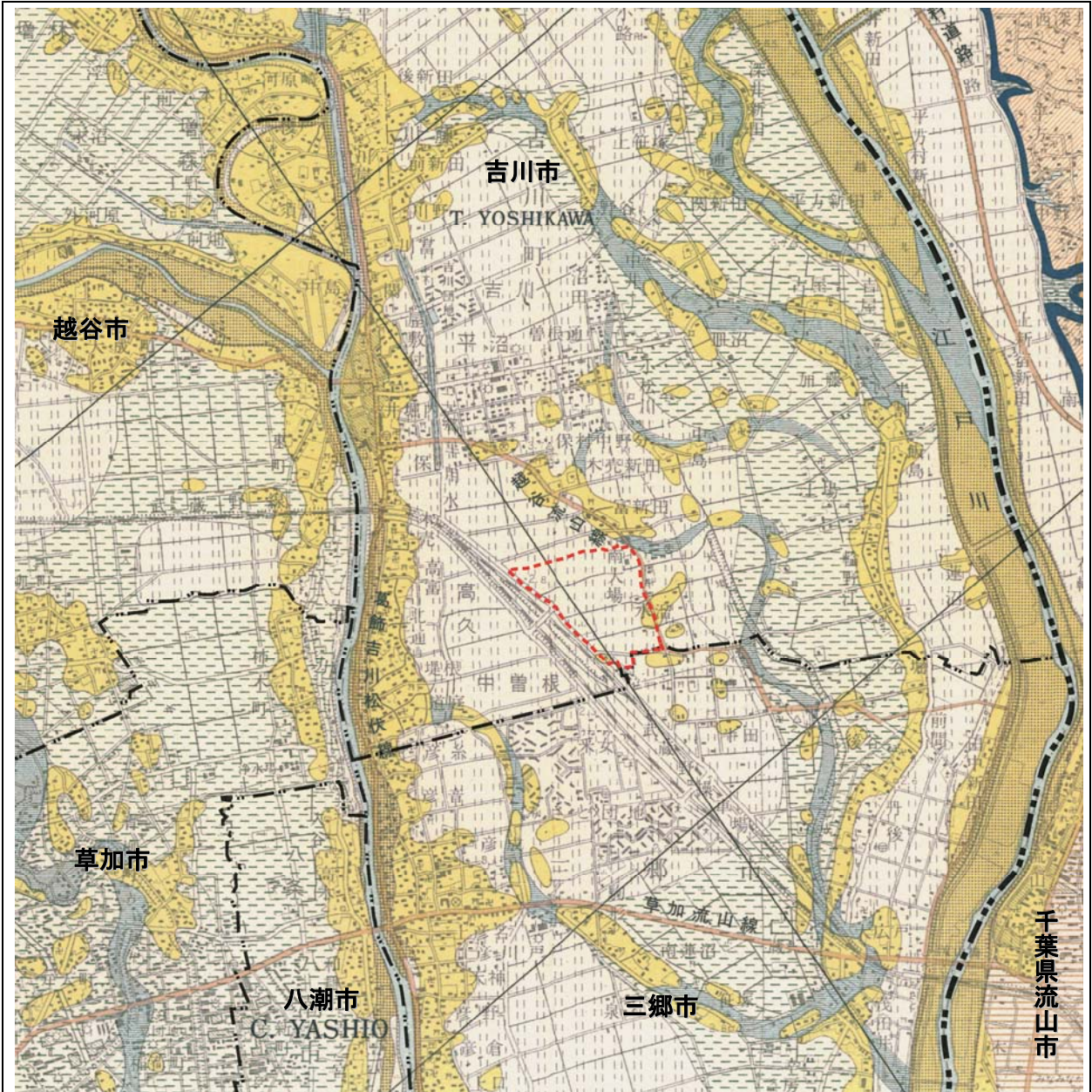
図 3-2-6 地形分類図
