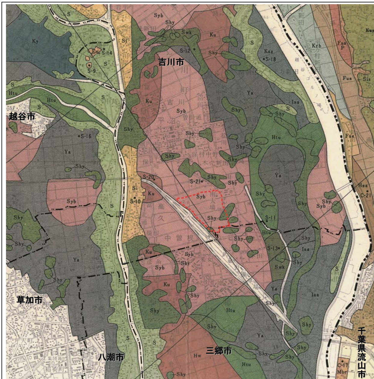
図 3-2-4 土壌図
