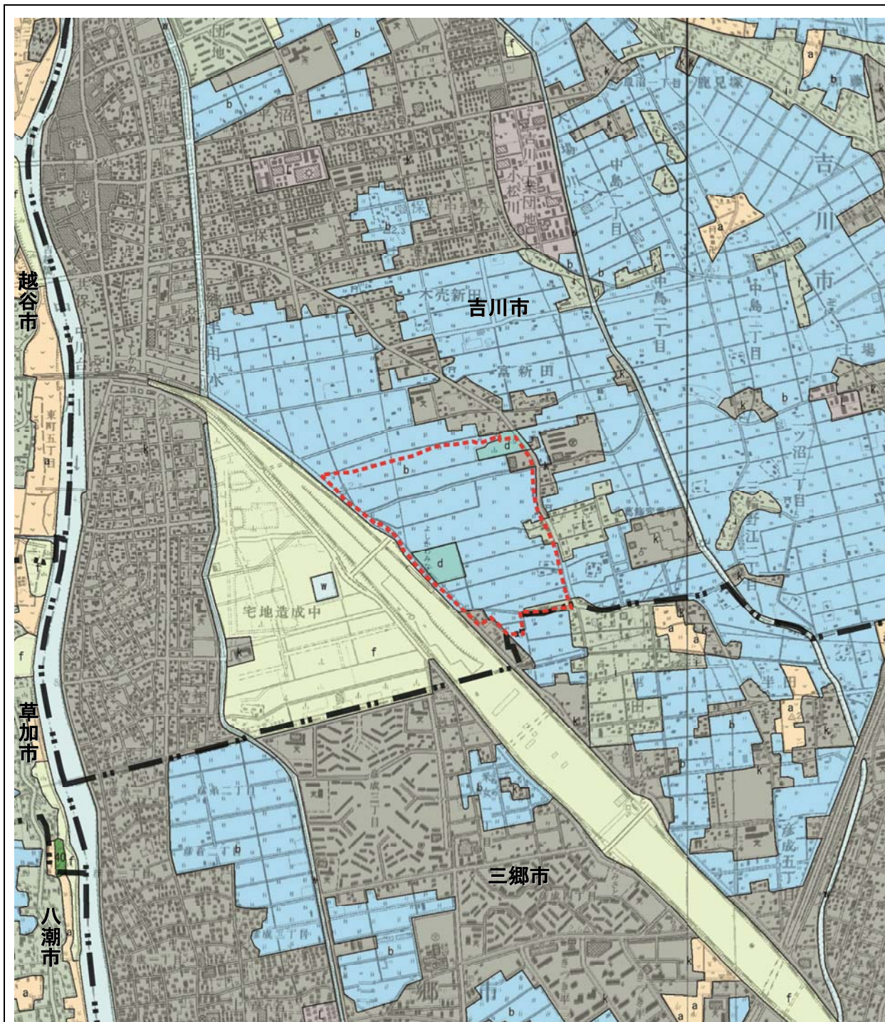
図 3-2-8 植生図
