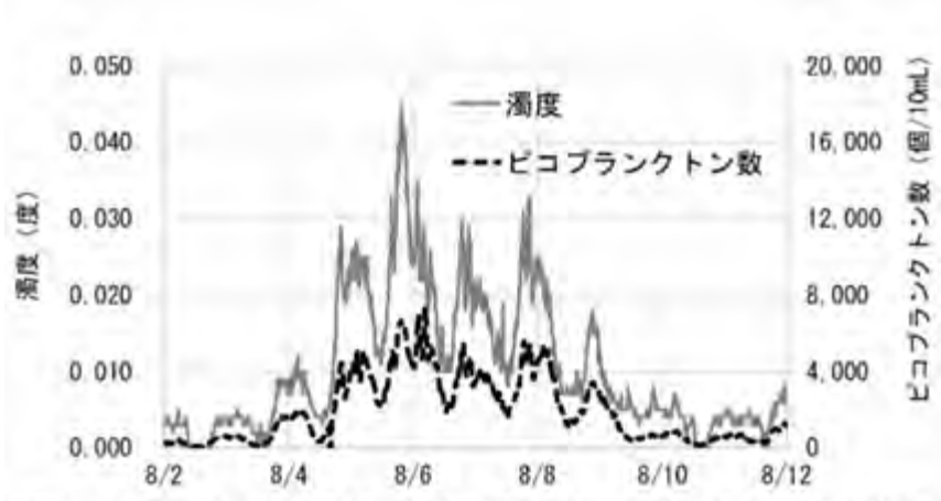
図 8－6－2 ろ過池出口水の濁度及びピコプランクトン数の推移（R5. 8. 2-12）
