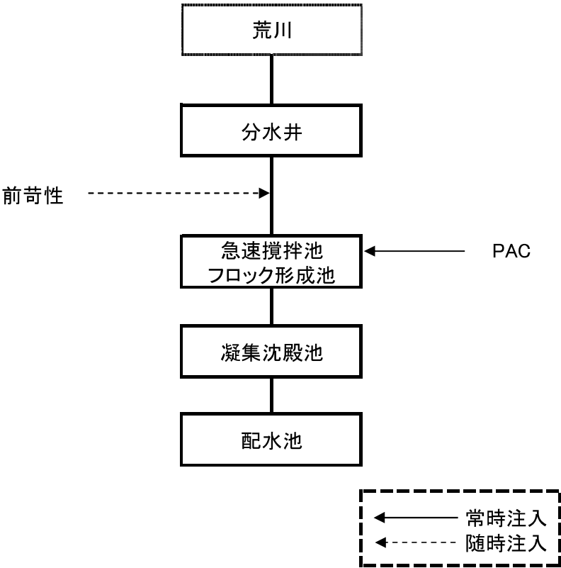
図 5－1 大久保浄水場の処理フロー
