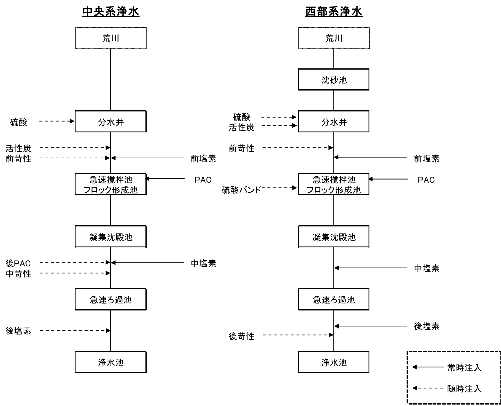
図 3－1－1 大久保浄水場 2 系統の処理フロー
