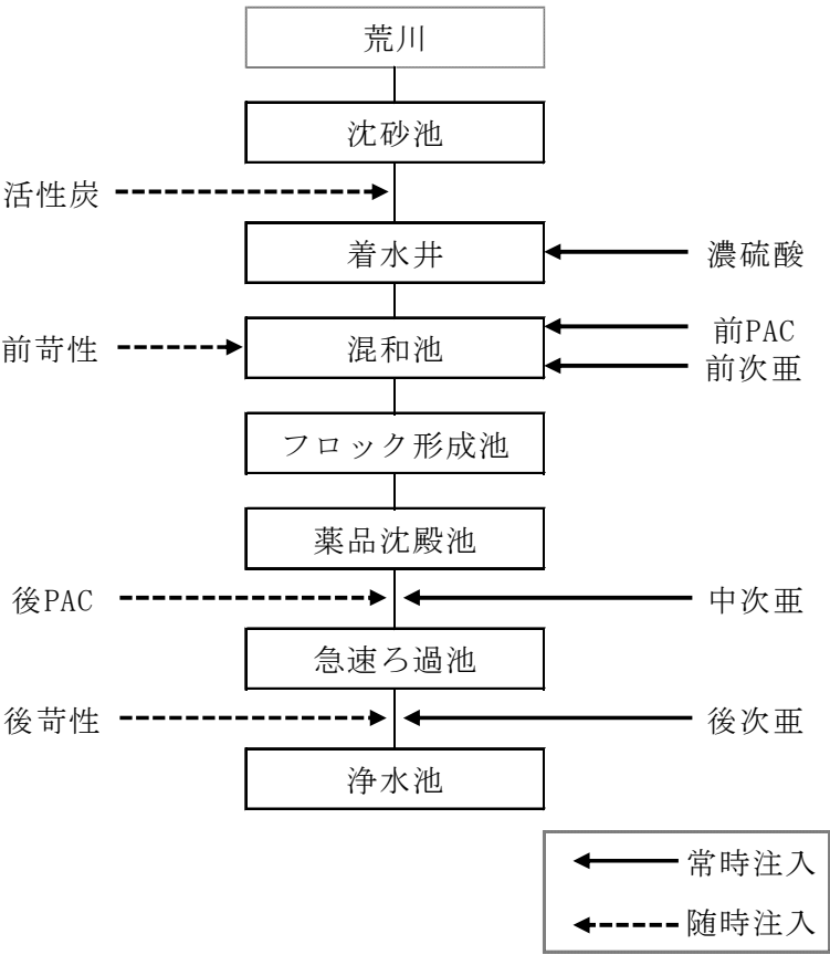
図3－5－1 吉見浄水場の処理フロー
