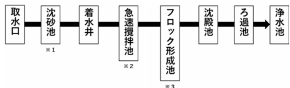
図 8－3－2 行田浄水場と大久保浄水場の浄水処理工程（概略）
