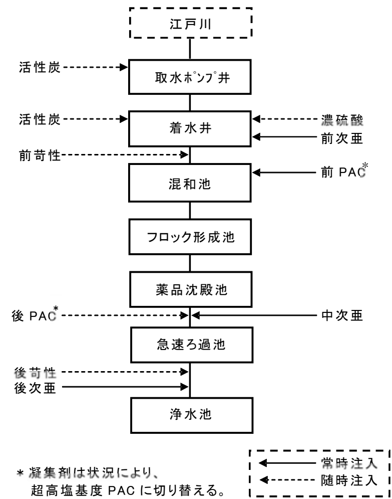
図 3－2－1 庄和浄水場の処理フロー
