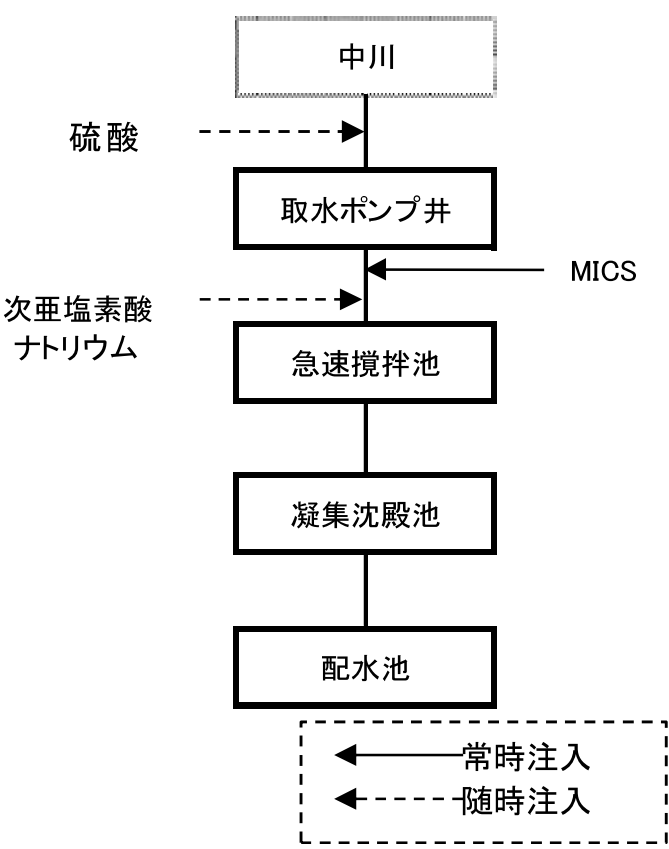
図 5－2－1 柿木浄水場の処理フロー
