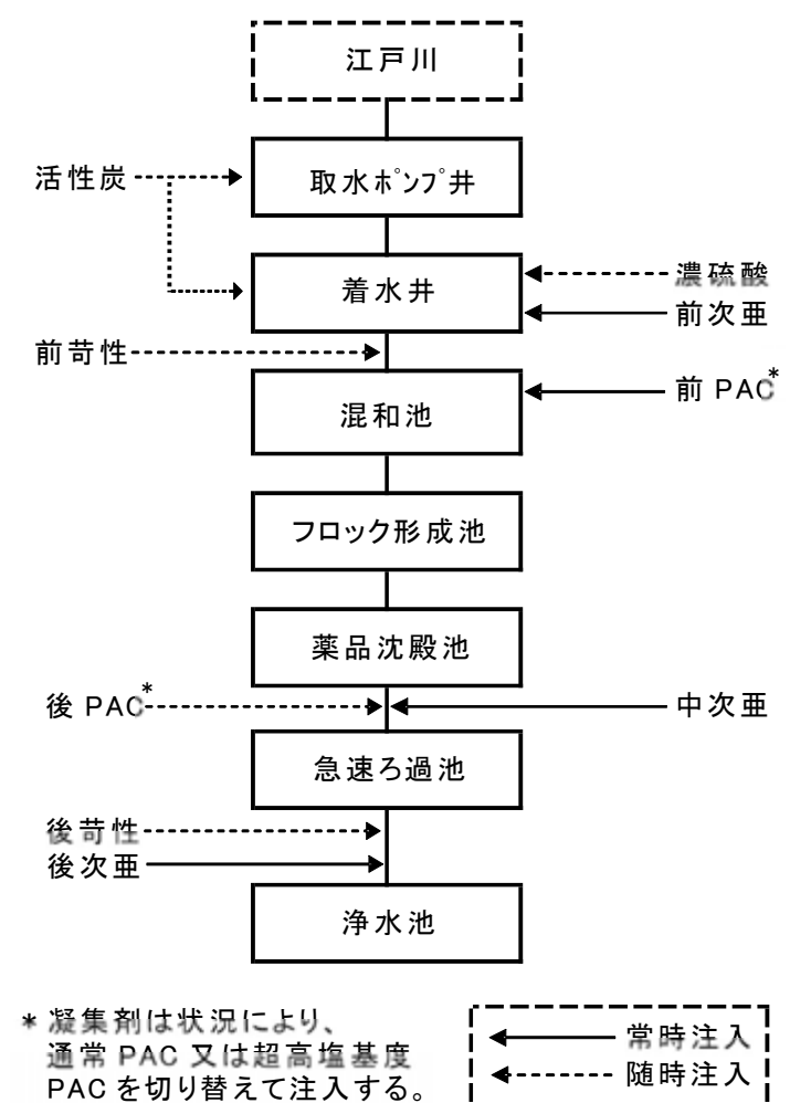
図 8-6-1 庄和浄水場の処理フロー
