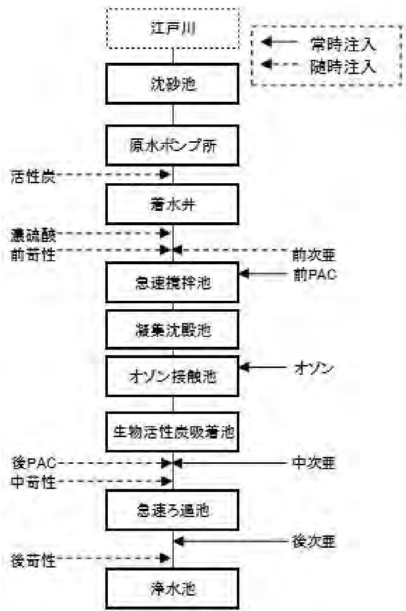
図 3－4－1 新三郷浄水場の処理フロー
