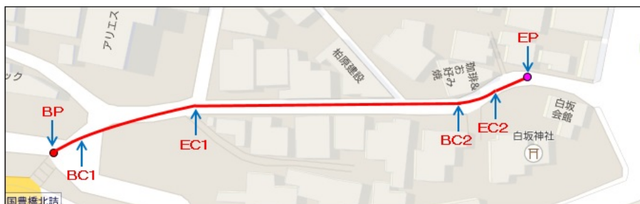
S字曲線の施工計画図
