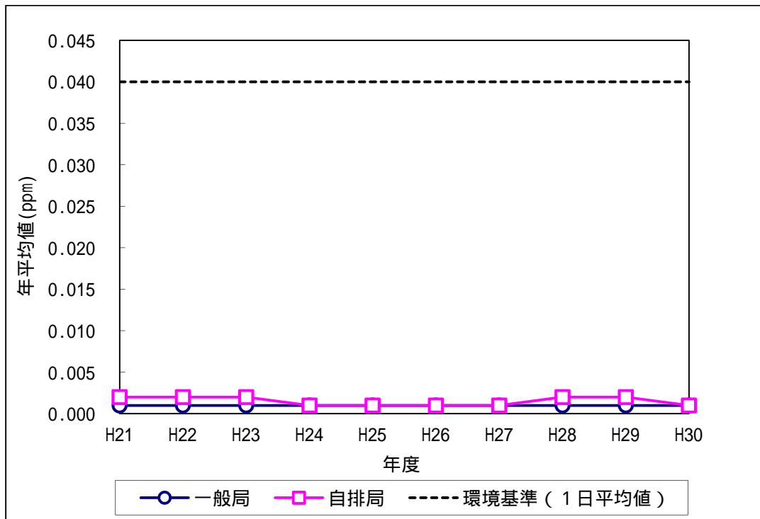
図1 二酸化硫黄の年平均値の推移グラフ(10年継続測定局)
