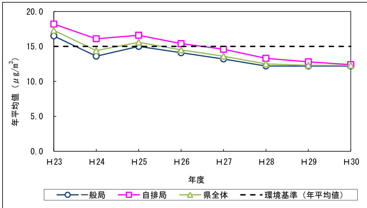
図 7 微小粒子状物質の年平均値の推移グラフ
