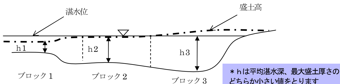
図-2-6 盛土行為に対する雨水流出抑制施設の容量の求め方
