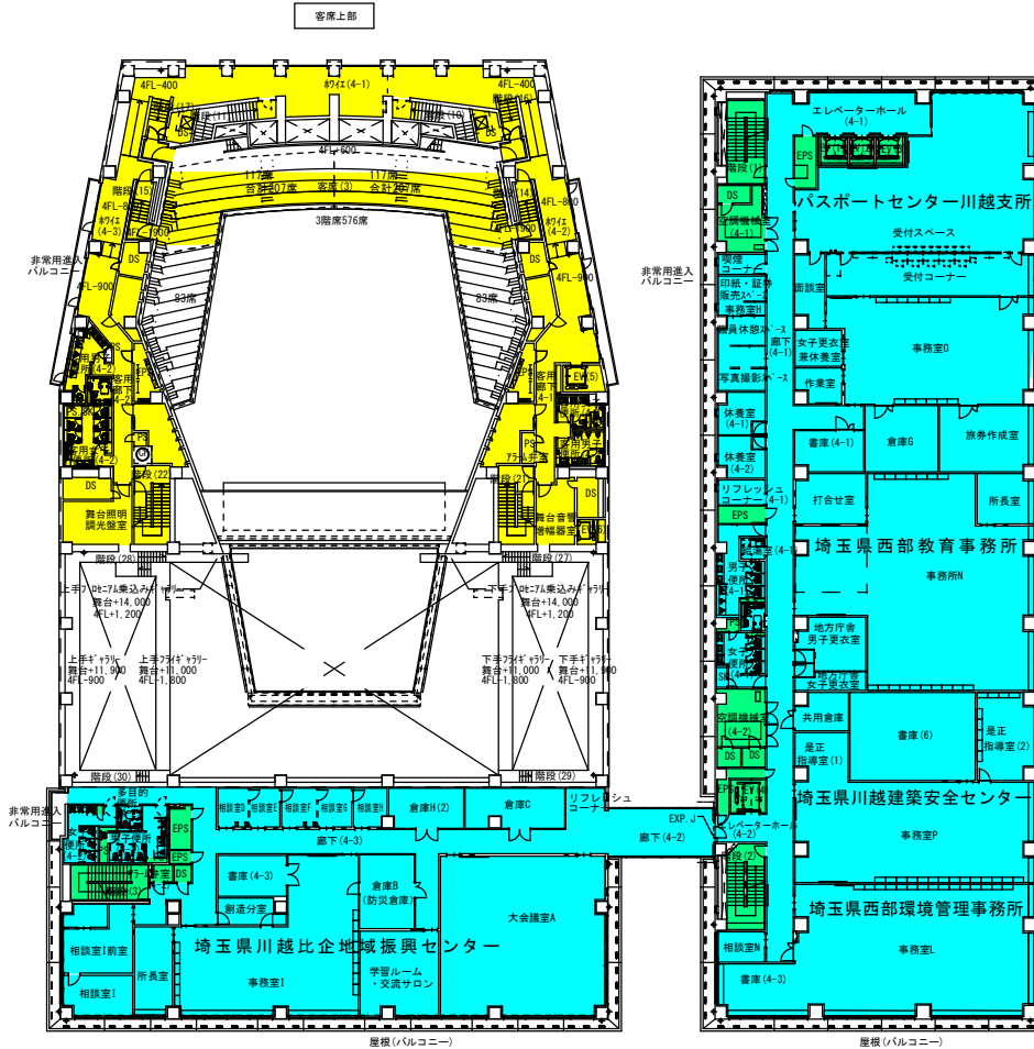
4階平面図 Scale:1/500
