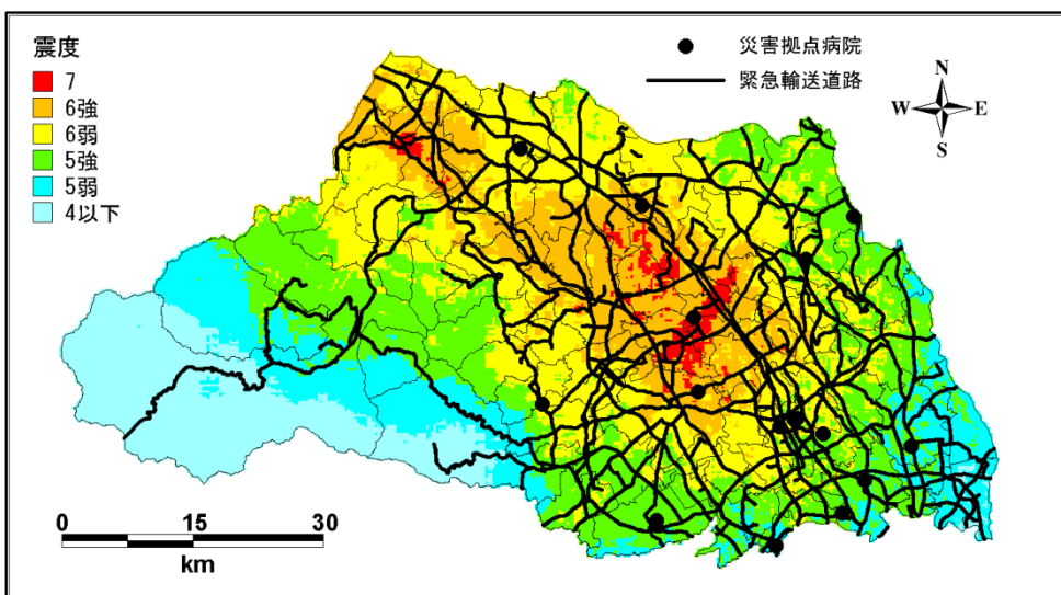
图 14.3-1(2) 災害拠点病院所在地周辺の震度分布図 (活断層型地震 関東平野北西縁断層帯地震)
