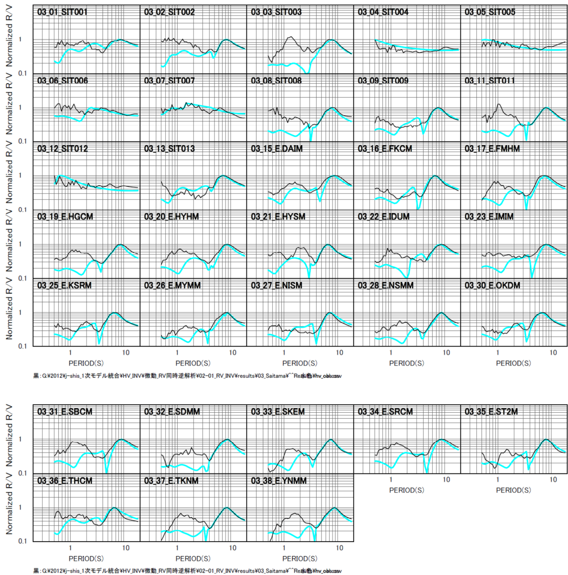
図 3. 1. 2-2(1) 観測 R/V スペクトルと理論 H/V スペクトルの比較 黒：観測 R/V スペクトル 水色：理論 H/V スペクトル
