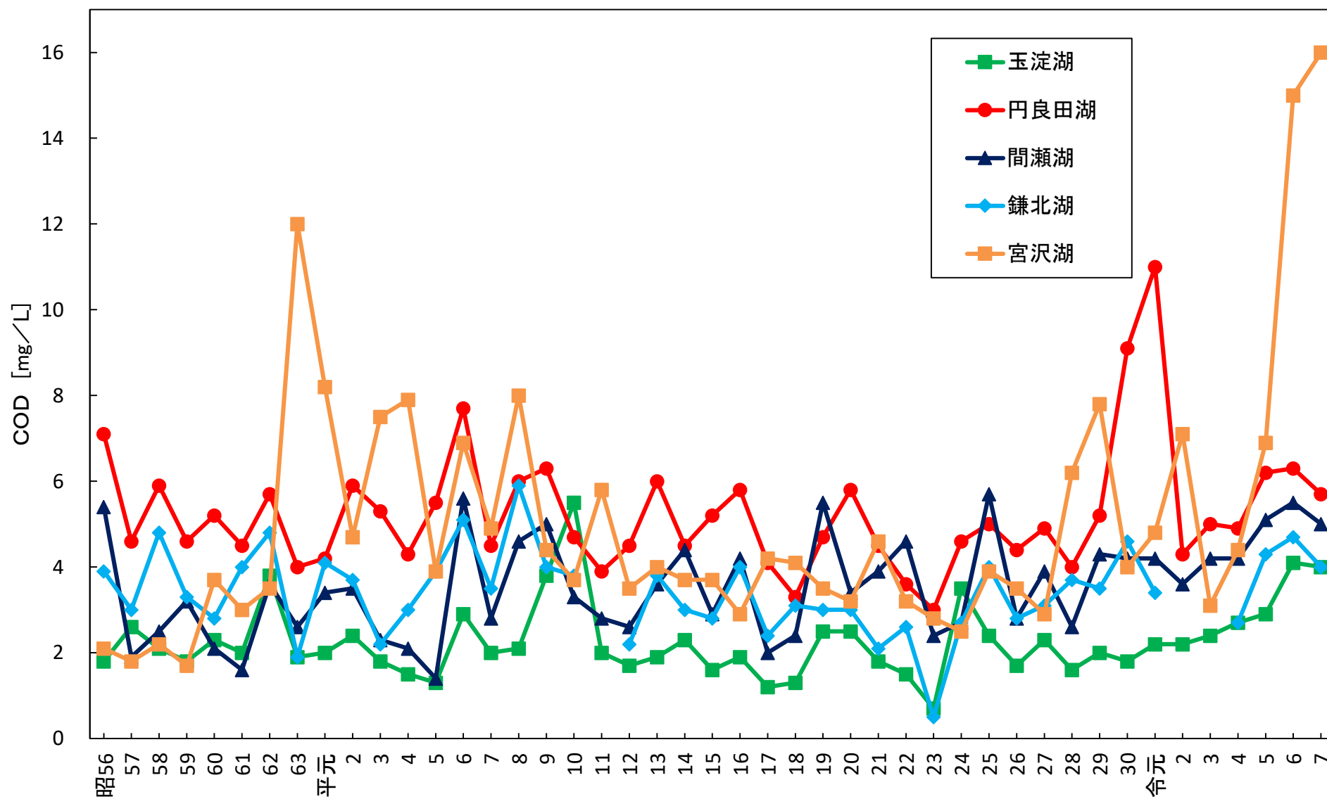
湖沼表層水のCOD経年変化（人工湖沼・夏季）
