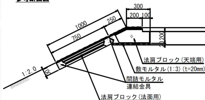
参考断面図
