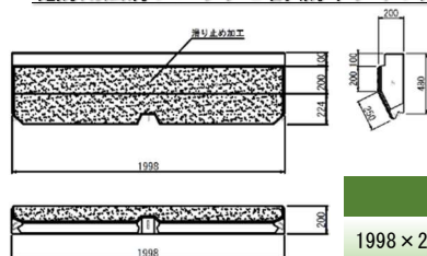
堤防用法肩ブロック 2 割(防草タイプ)
