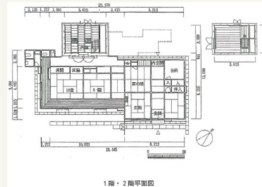
1階・2階平面図
