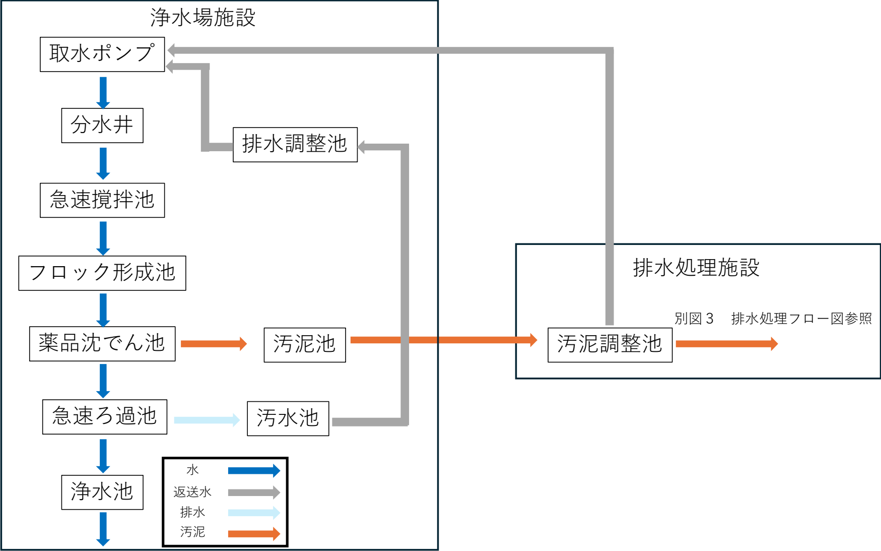
別図2 大久保浄水場排水処理フロー図
