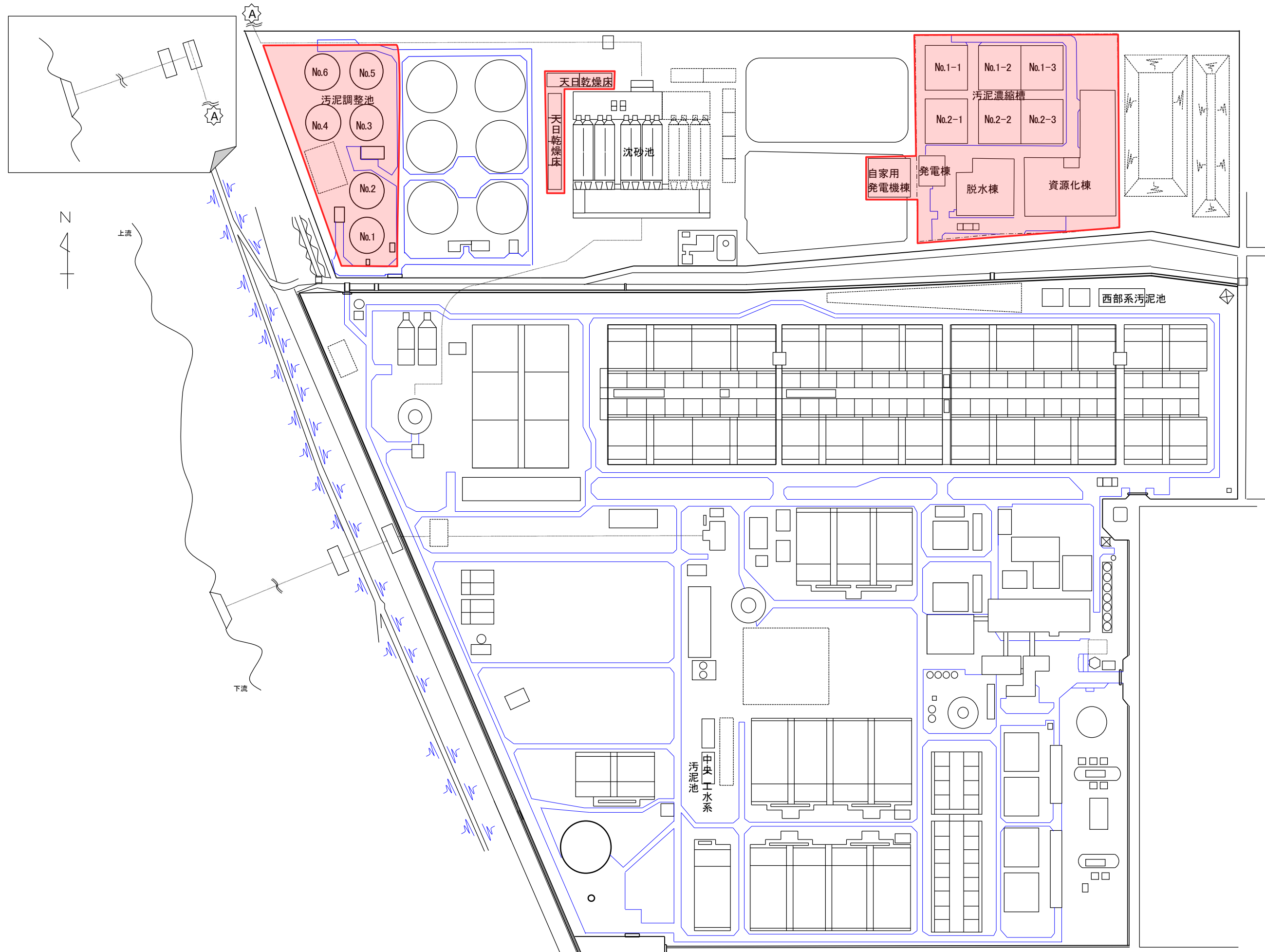
別図1 大久保浄水場全体平面図
