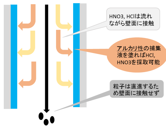
図1 デニューダ法の原理
