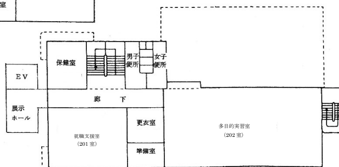
2階平面図
