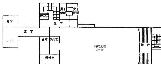
5階平面図
