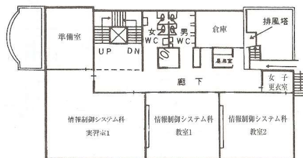
2階平面図
