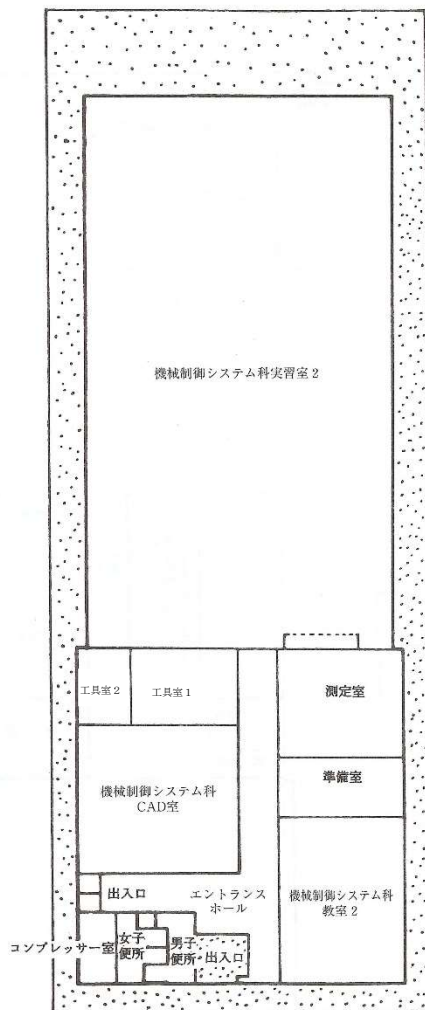
平面図
