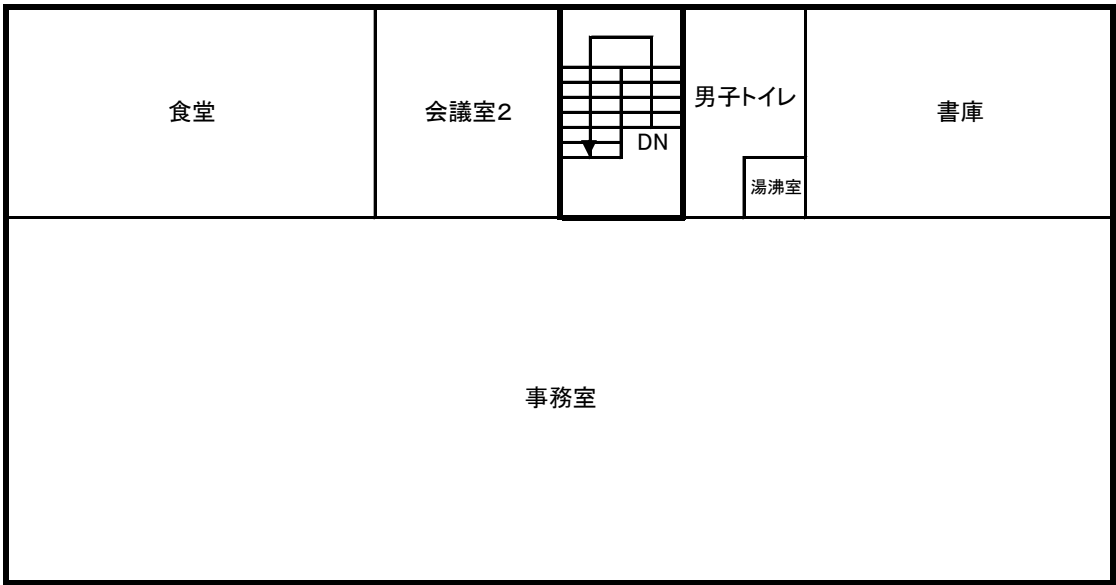
2階平面図
