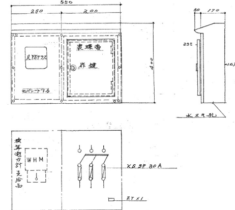
動力引込開閉器箱図 屋外防水型
