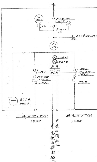
動力操作盤接続図及操作回路図
