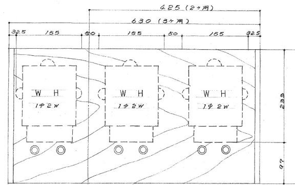
電灯用積算配電盤配置図
