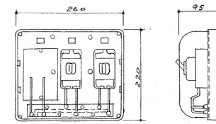
NFB 2ヶ用反3ヶ用 配電用電灯分盤詳細図
