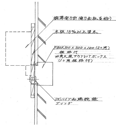
電灯用積算配電盤配置図
