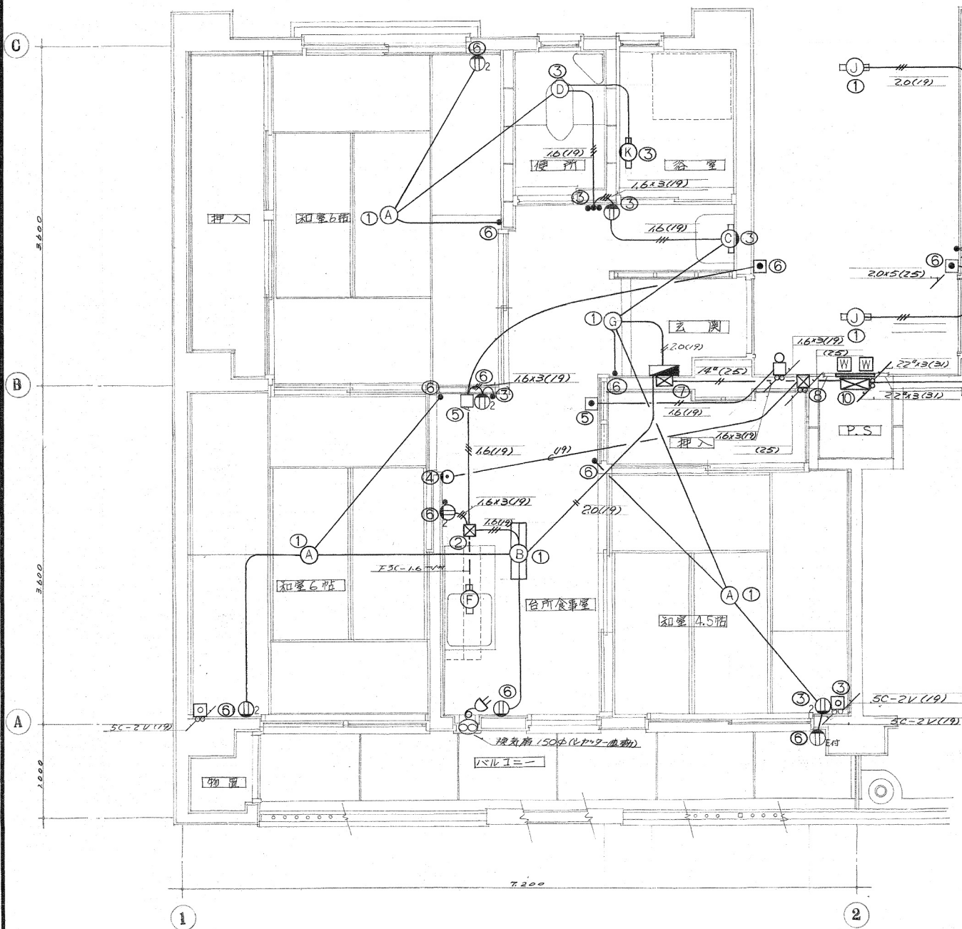
平面詳細図 1/30
