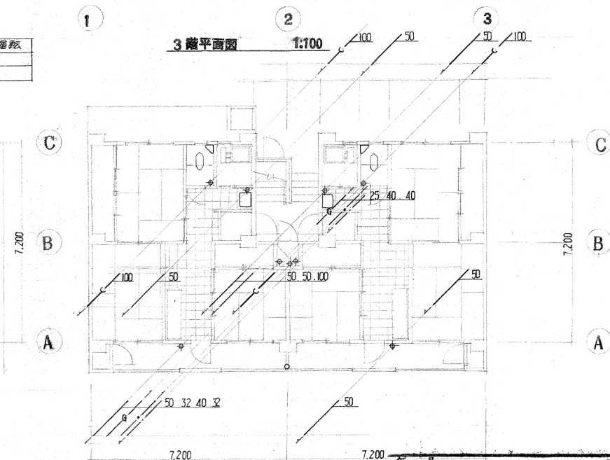
2 階平面図 1:100
