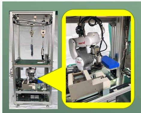
部品検査等 簡易作業等を行う 「セルロボット」 ヤマヤE&S株式会社 (本社：熊谷市)
