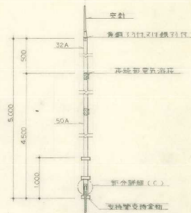
避雷針取付詳細図 (屋付型)
