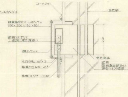
端子箱取付 詳細図
