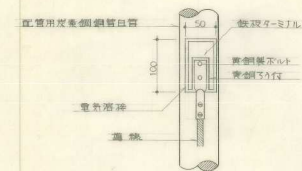
部分詳細 (C)
