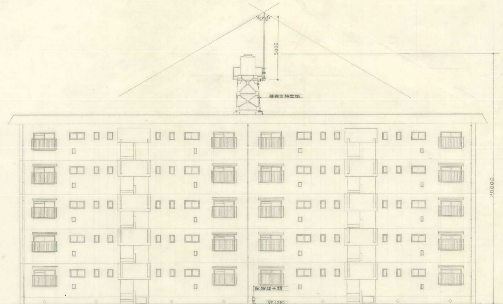
北立面図 1:100
