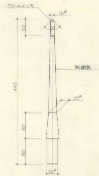
避雷針 B型
