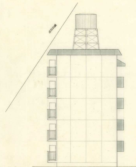
南側立面図
