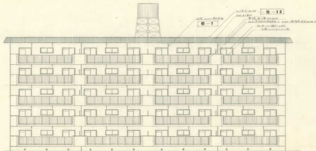
西側立面図
