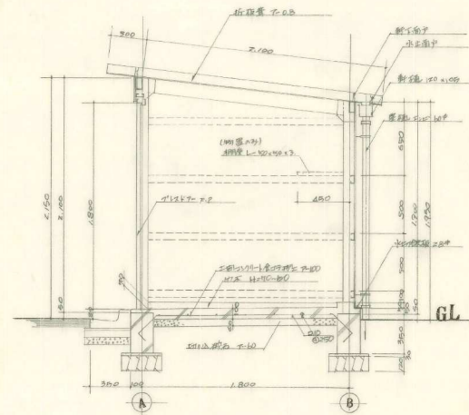
断面図 S=1:20
