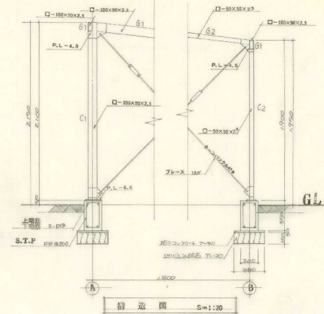
断面図 S=1:20
