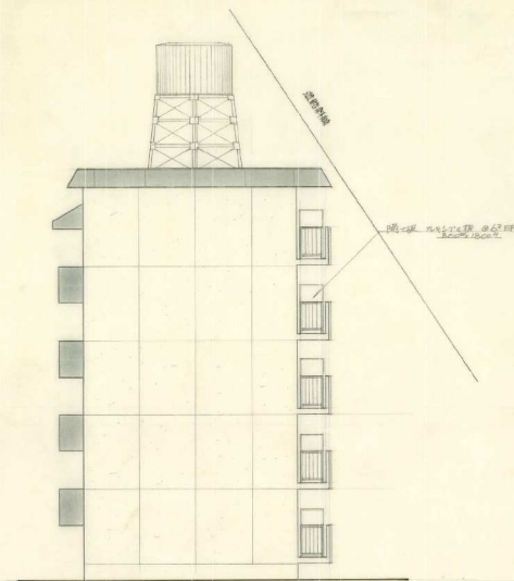
北側立面図
