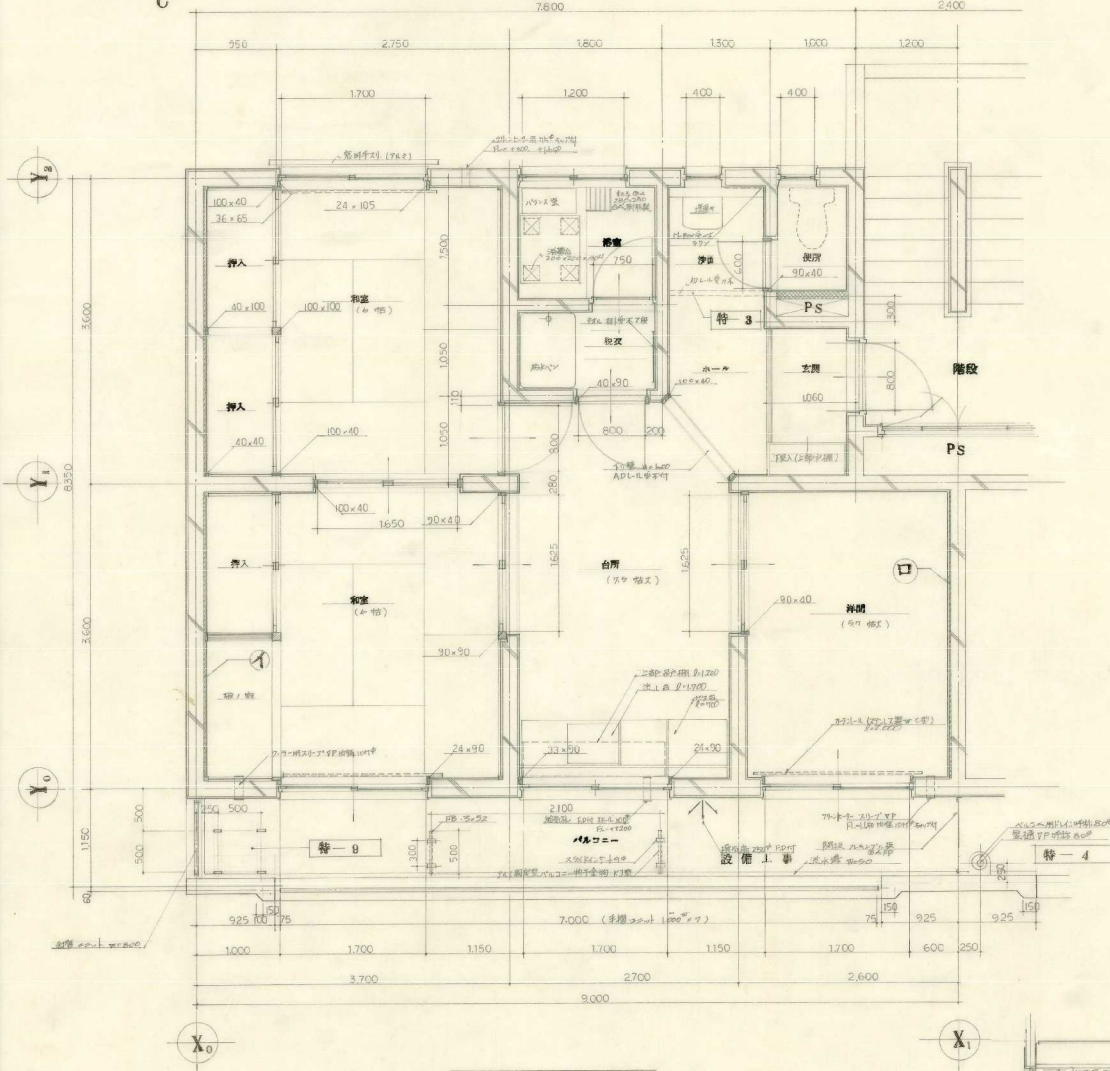
平面詳細図 S=1:30
