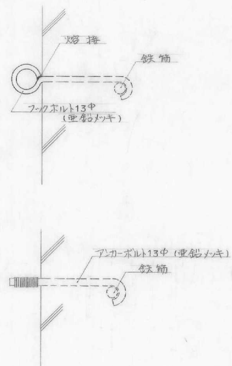
フックボルト、アンカーボルト取付略図
