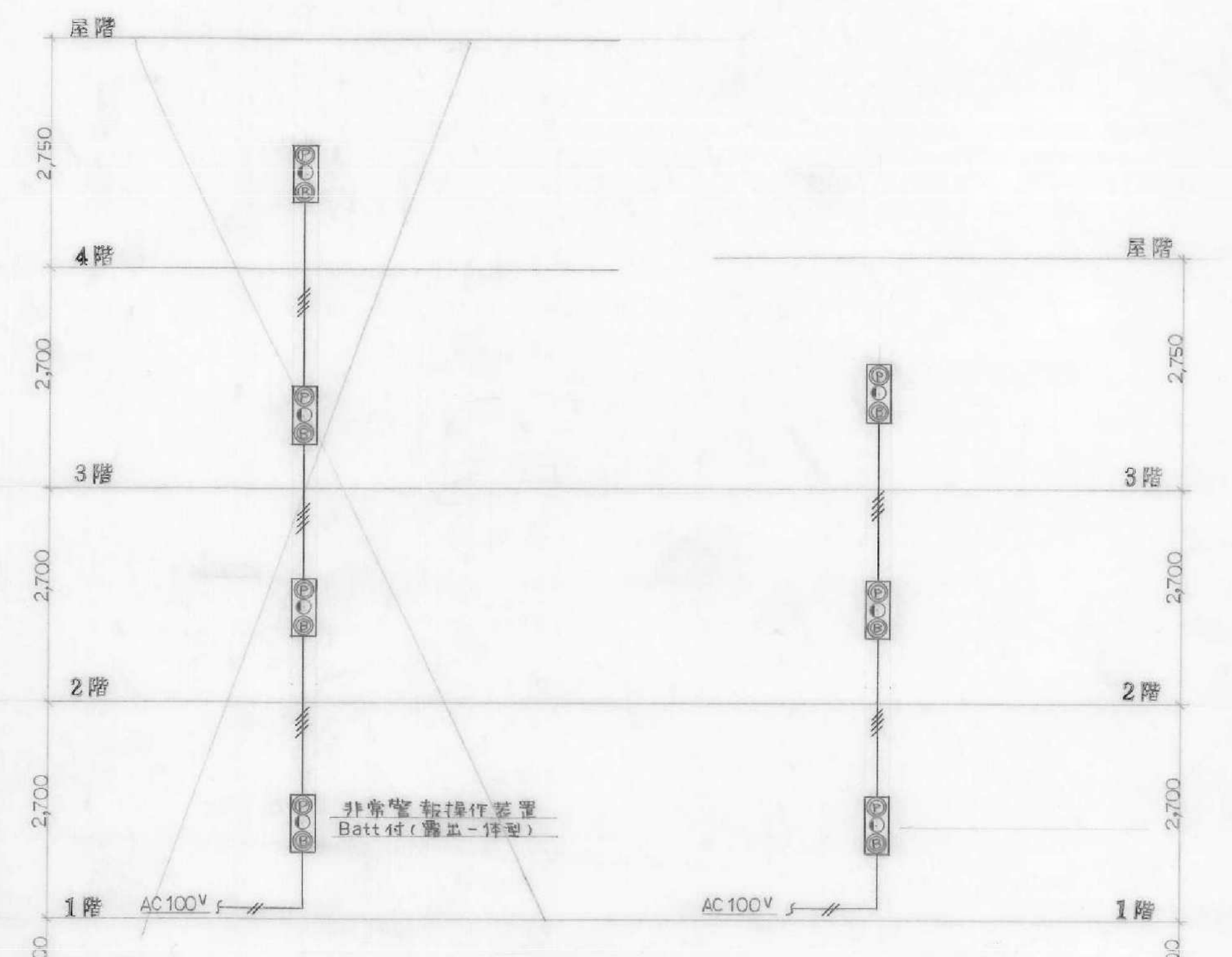
非常警報 設備系統図
