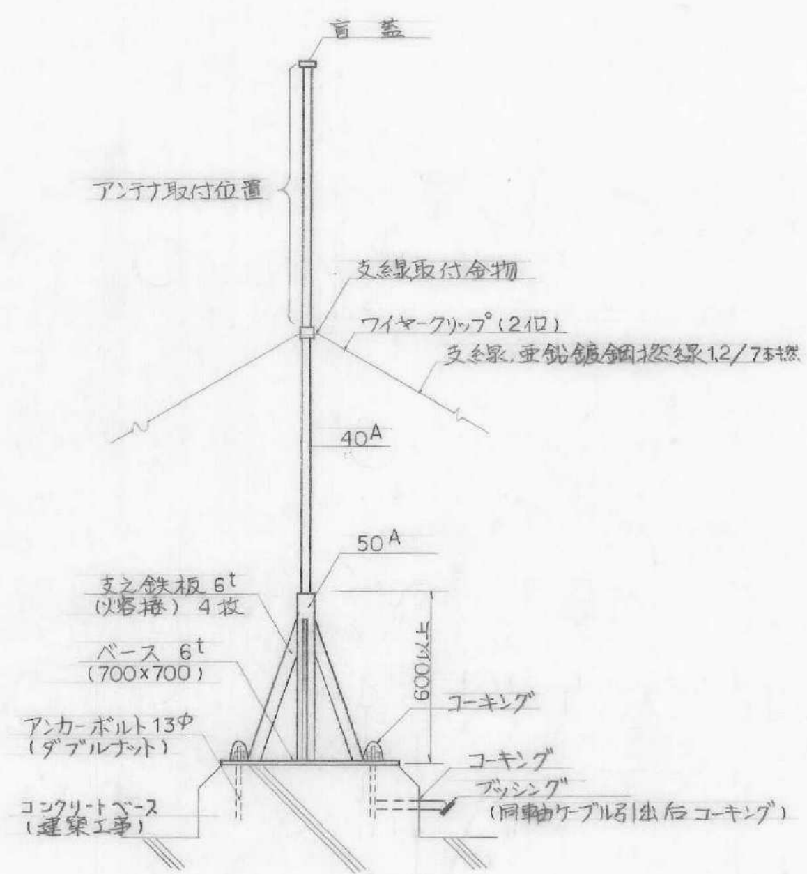
アンテナマスト取付詳細図 (NO SCALE)
