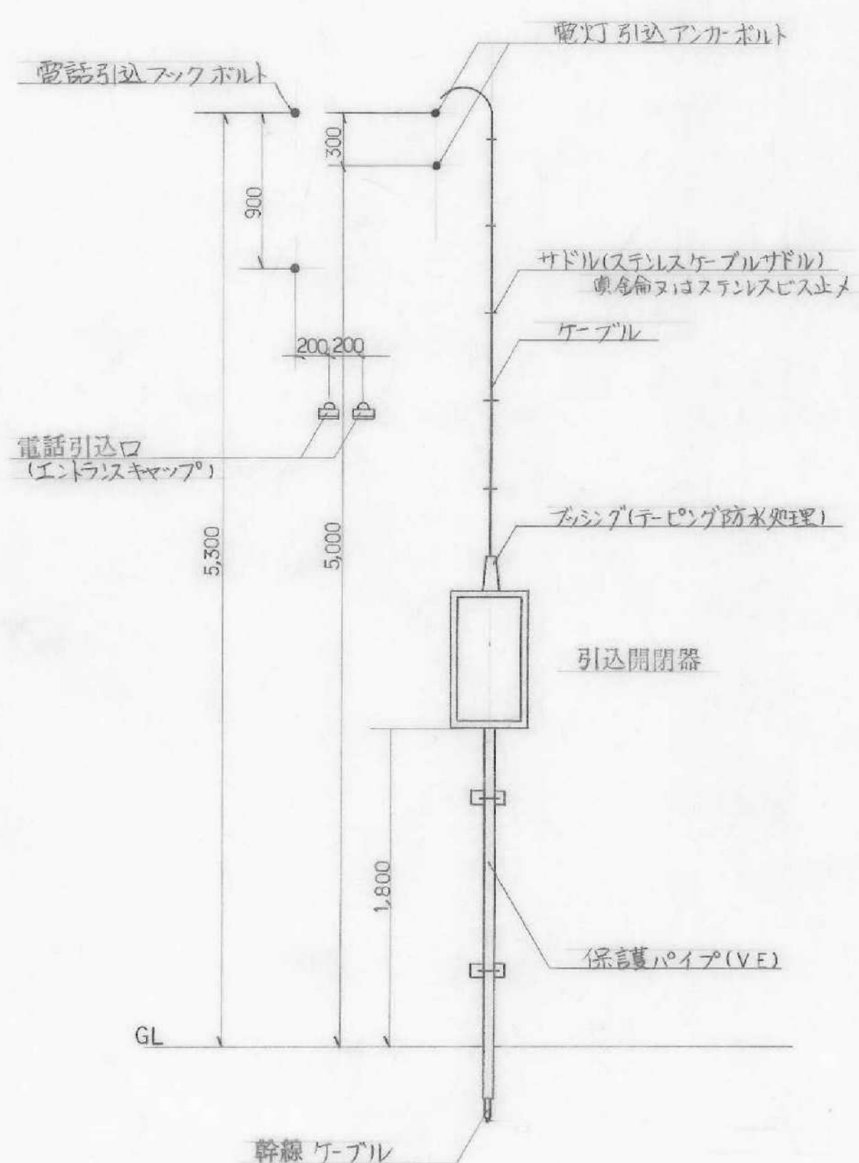
引込線(引込線)配線略図
