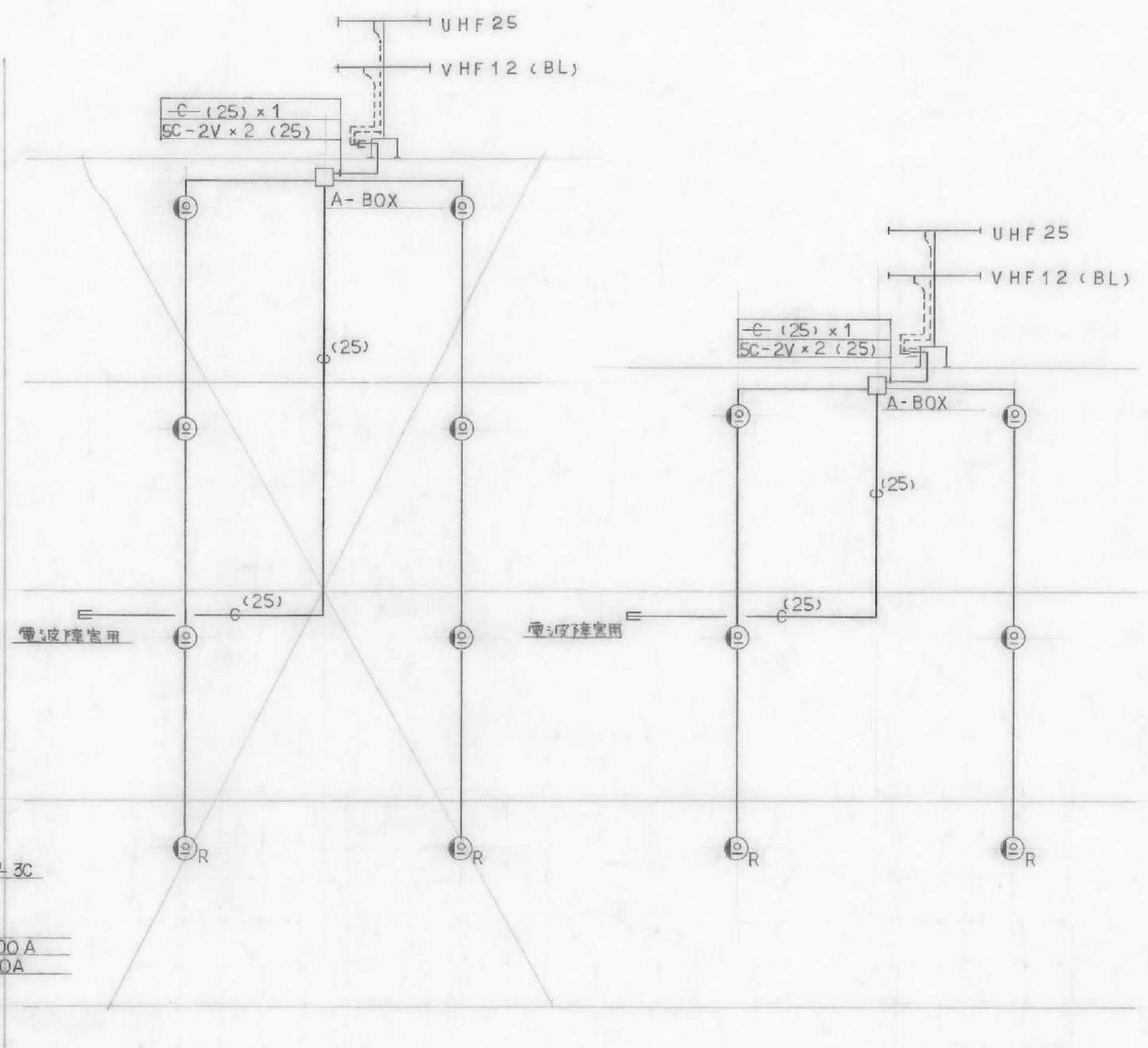
テレビ共同視聴 設備系統図
