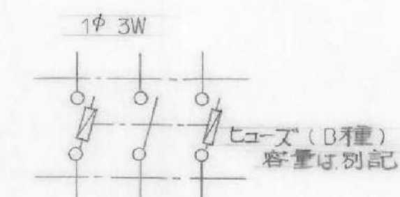
結線図
