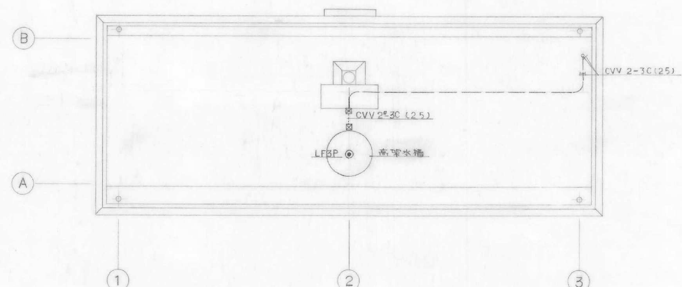
屋階 平面図 S=1:100
