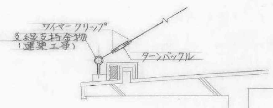
支線取付側面図 (NO SCALE)
