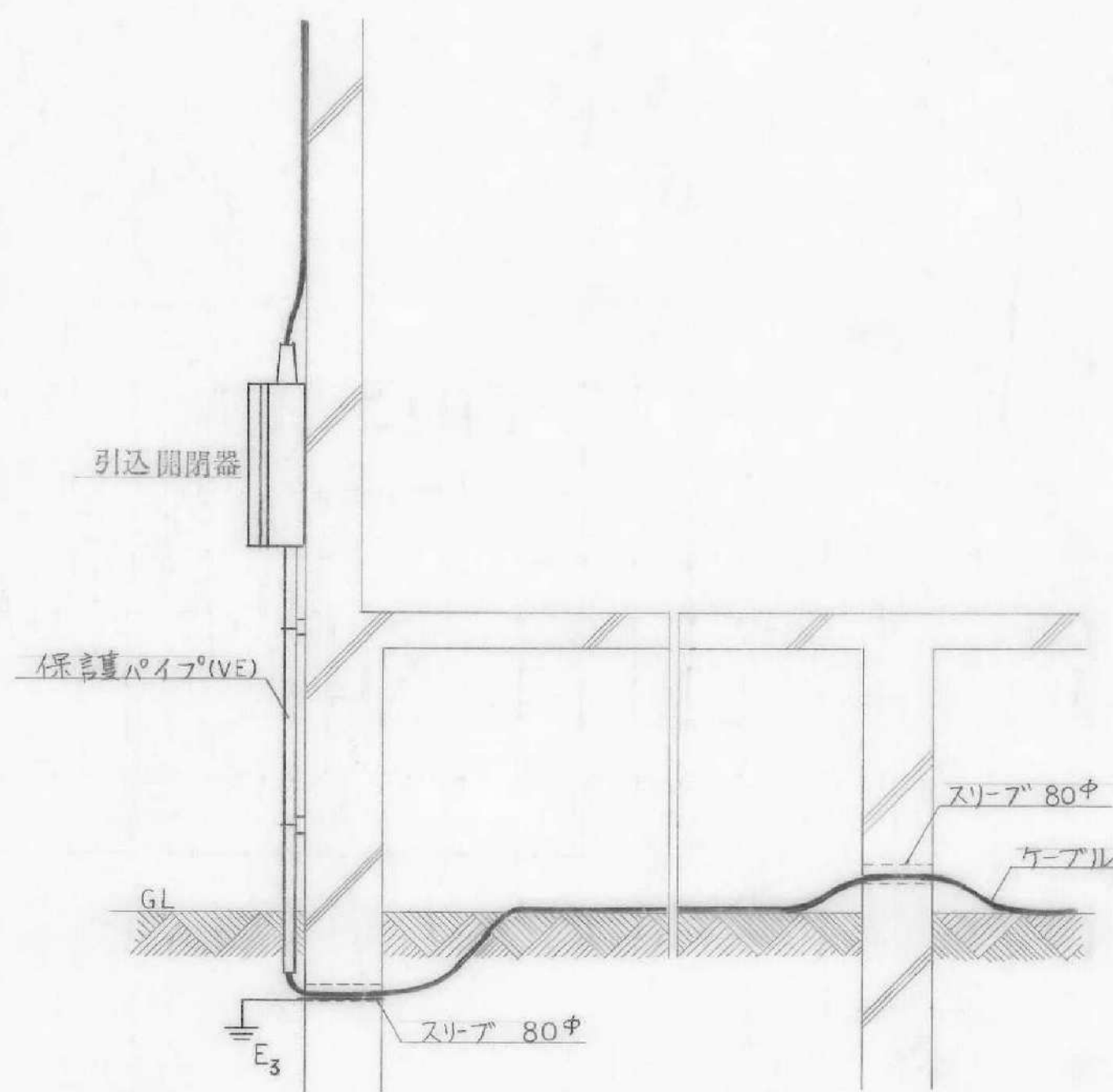
引込口断面図
