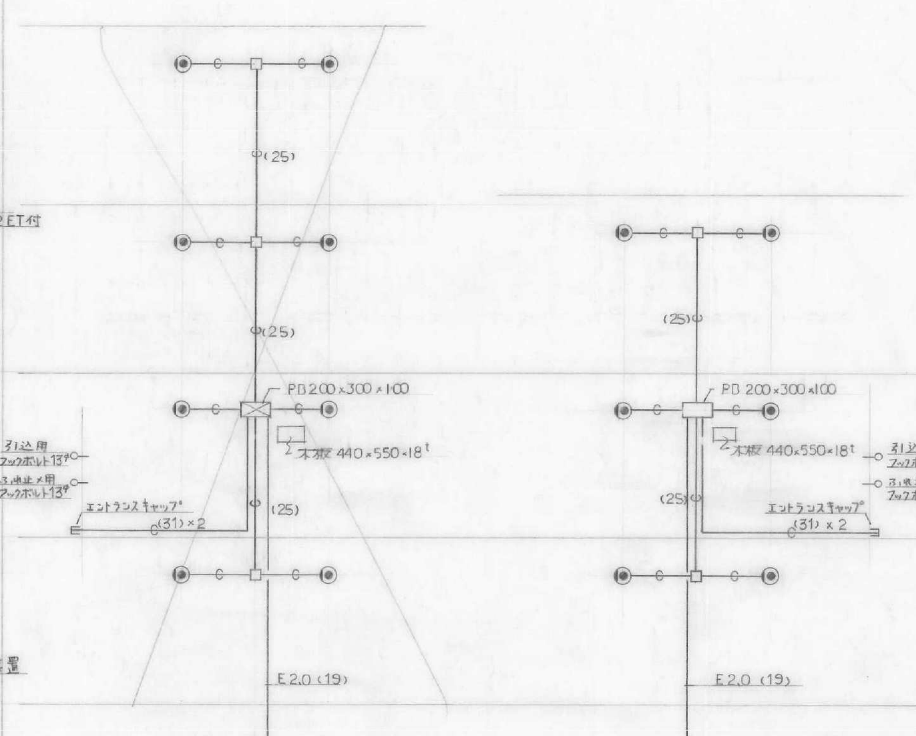
電話 配管 設備系統図
