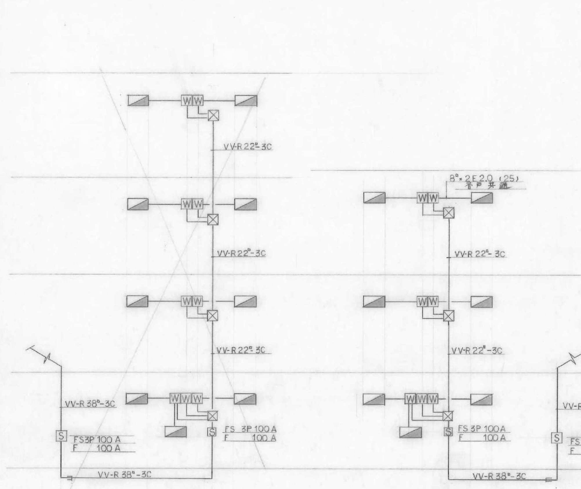
電灯 系統図
