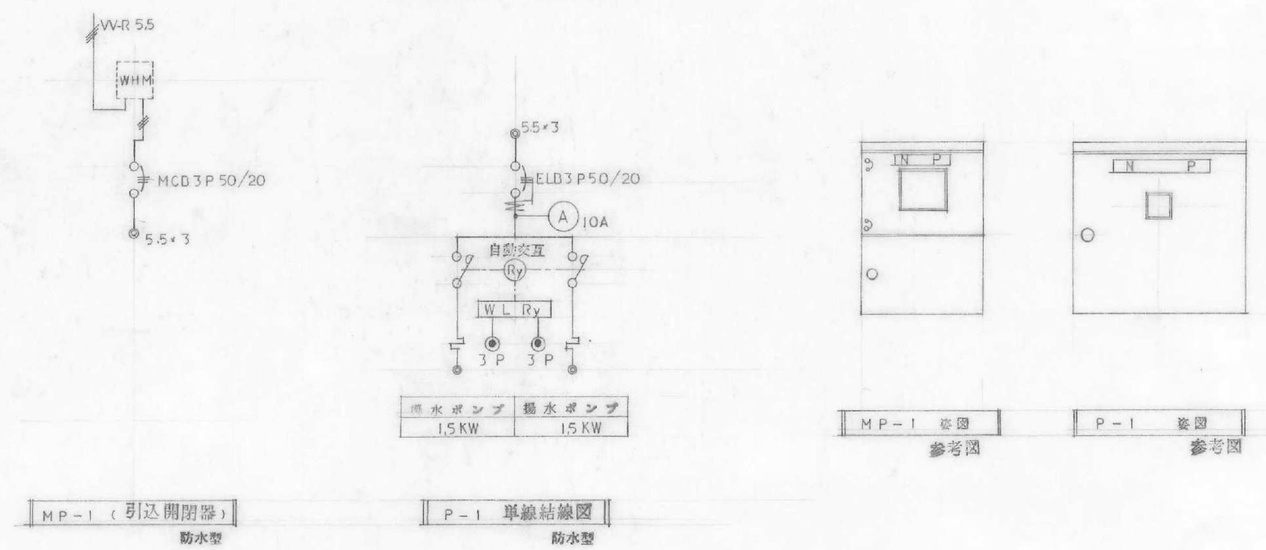
動力設備系統図
