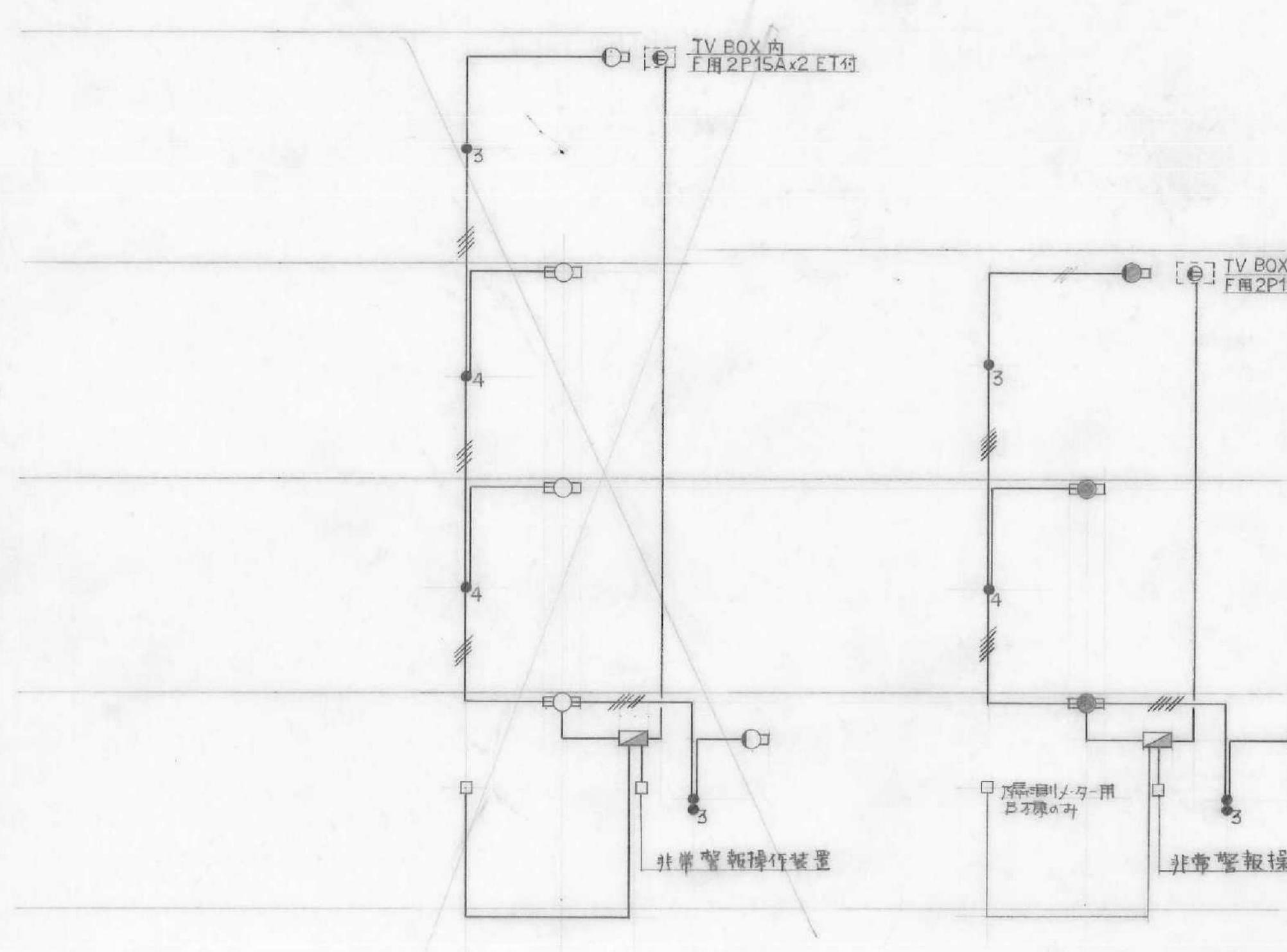
共用灯 系統図
