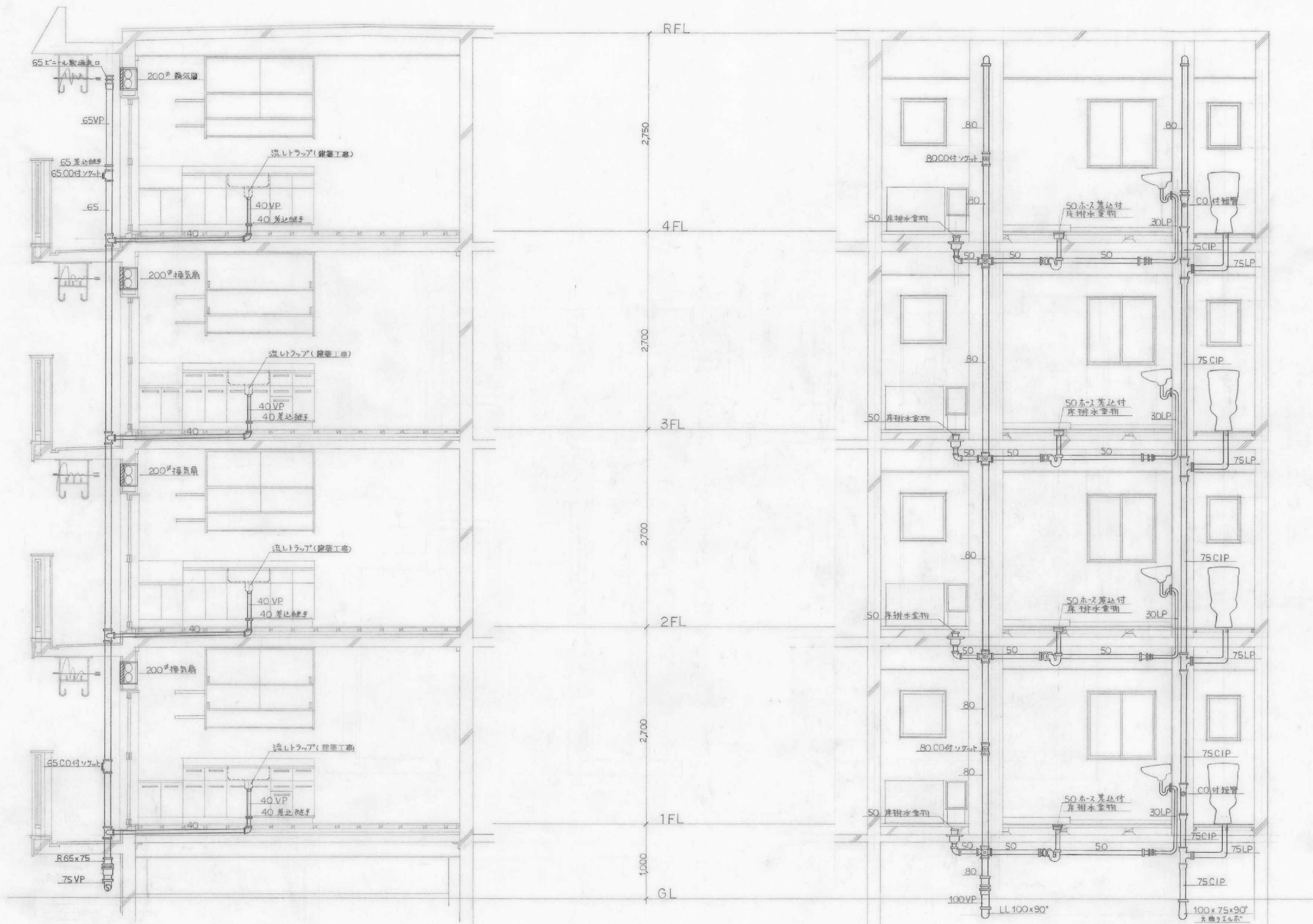
流シ排水立管詳細図 S=1:30
