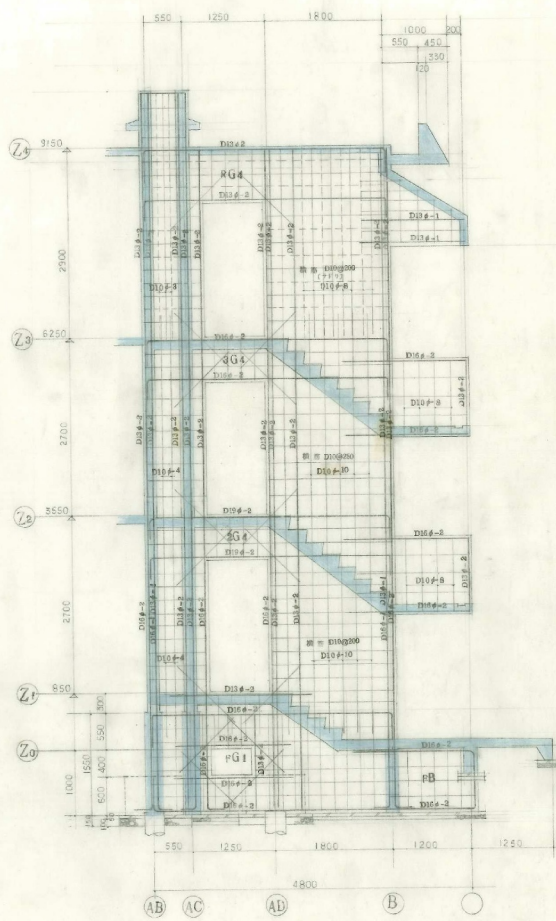
階段部断面 S 1:40
