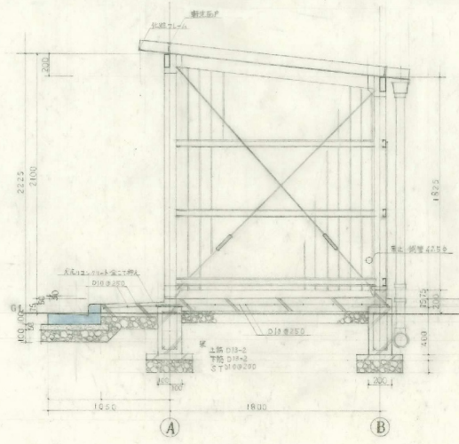
①通信組図詳細図 S 1:20
