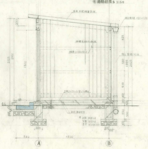
②通信組図詳細図 S 1:20
