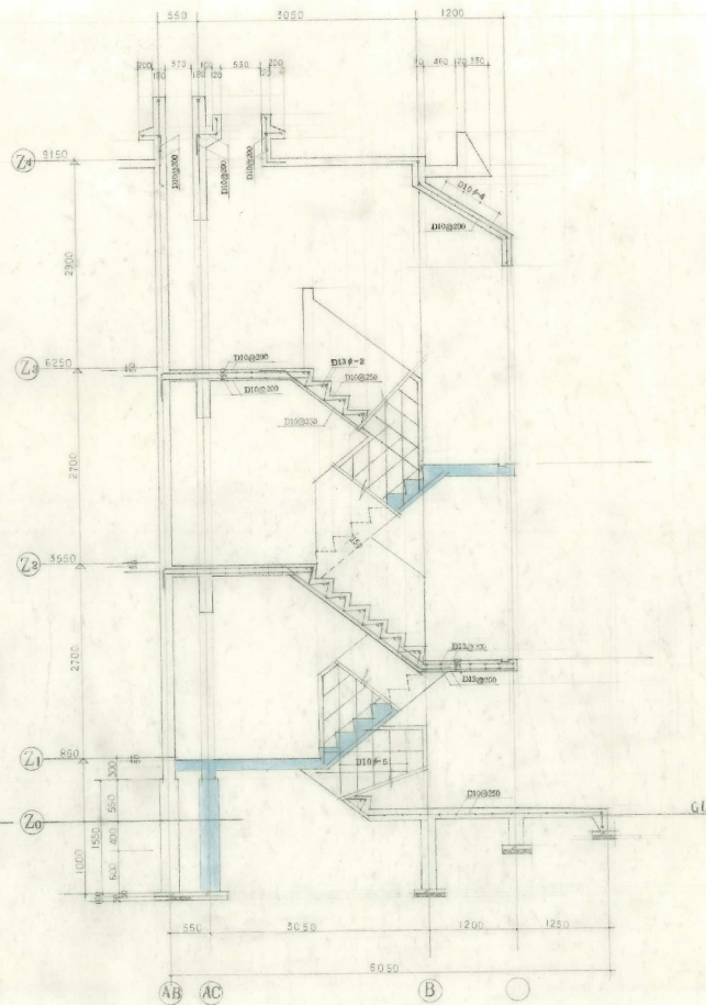
階段部断面 S 1:40
