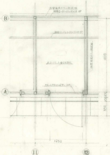
平面詳細図 S 1:20
