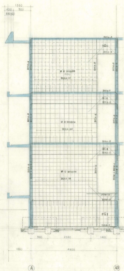
2F 通稱組圖 S 1:40
