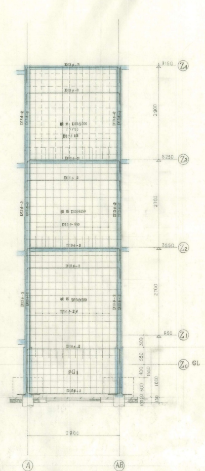
3F 通稱組圖 S 1:40
