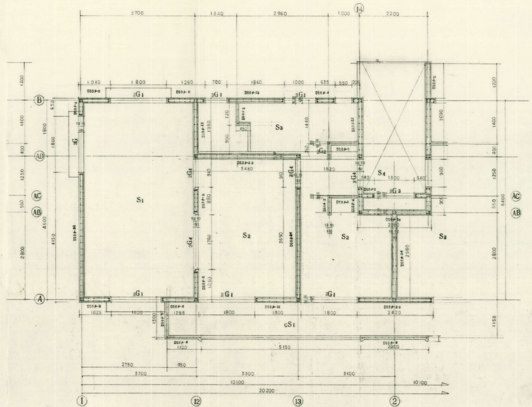
1階平面配筋図 S 1:140 (見上図)
