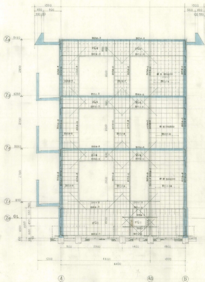
1F 通稱組圖 S 1:40
