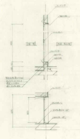
戸窓台部断面図 S 1:20
