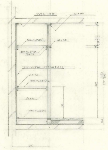
戸窓台部断面図 S 1:20
