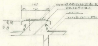
戸窓台部断面図 S 1:30
