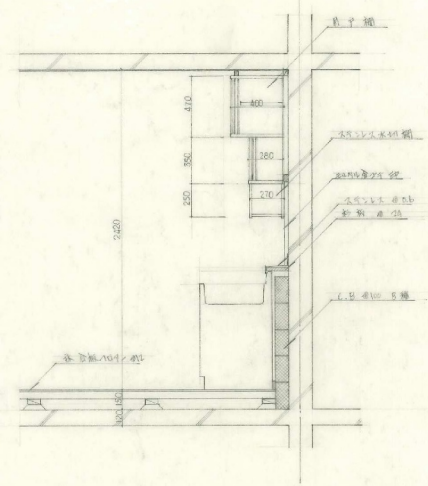
戸窓台部断面図 S 1:20
