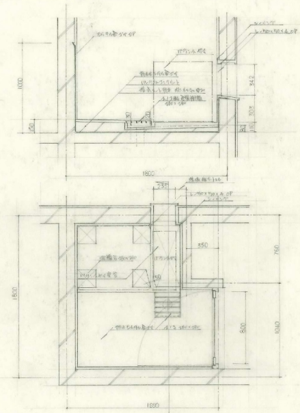
戸窓台部断面図 S 1:20
