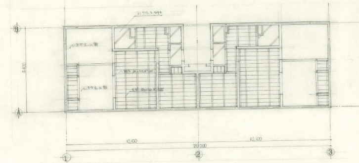
2F 平面図 S 1:100
