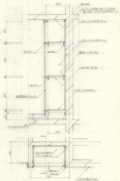
戸窓台部断面図 S 1:20
