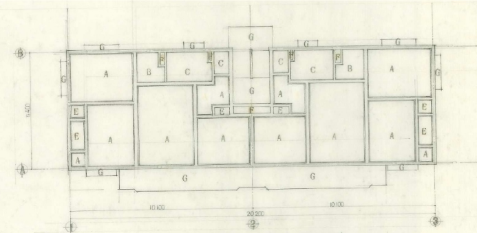
5F 平面図 S 1:100
