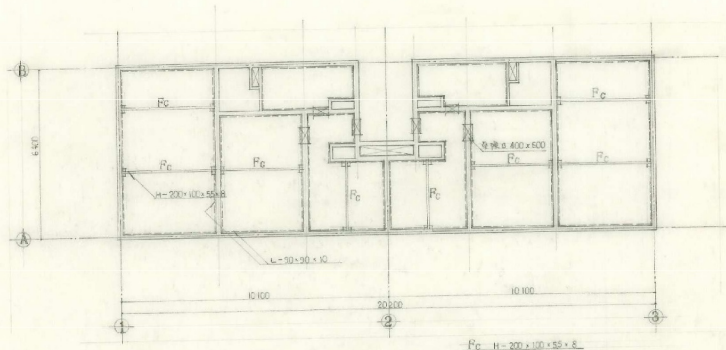
1F 平面図 S 1:100
