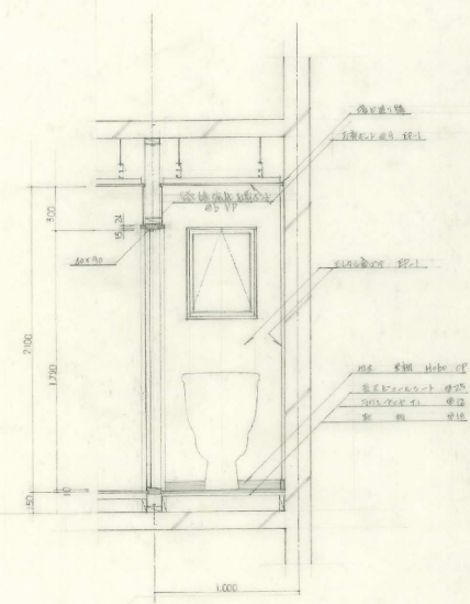
戸窓台部断面図 S 1:20
