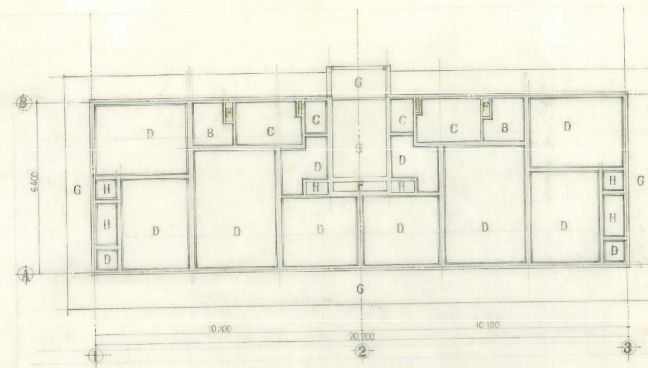
4F 平面図 S 1:100
