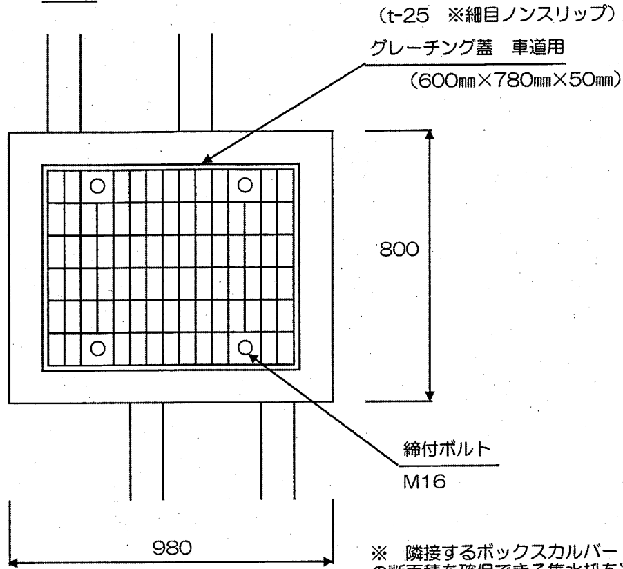
平面図
