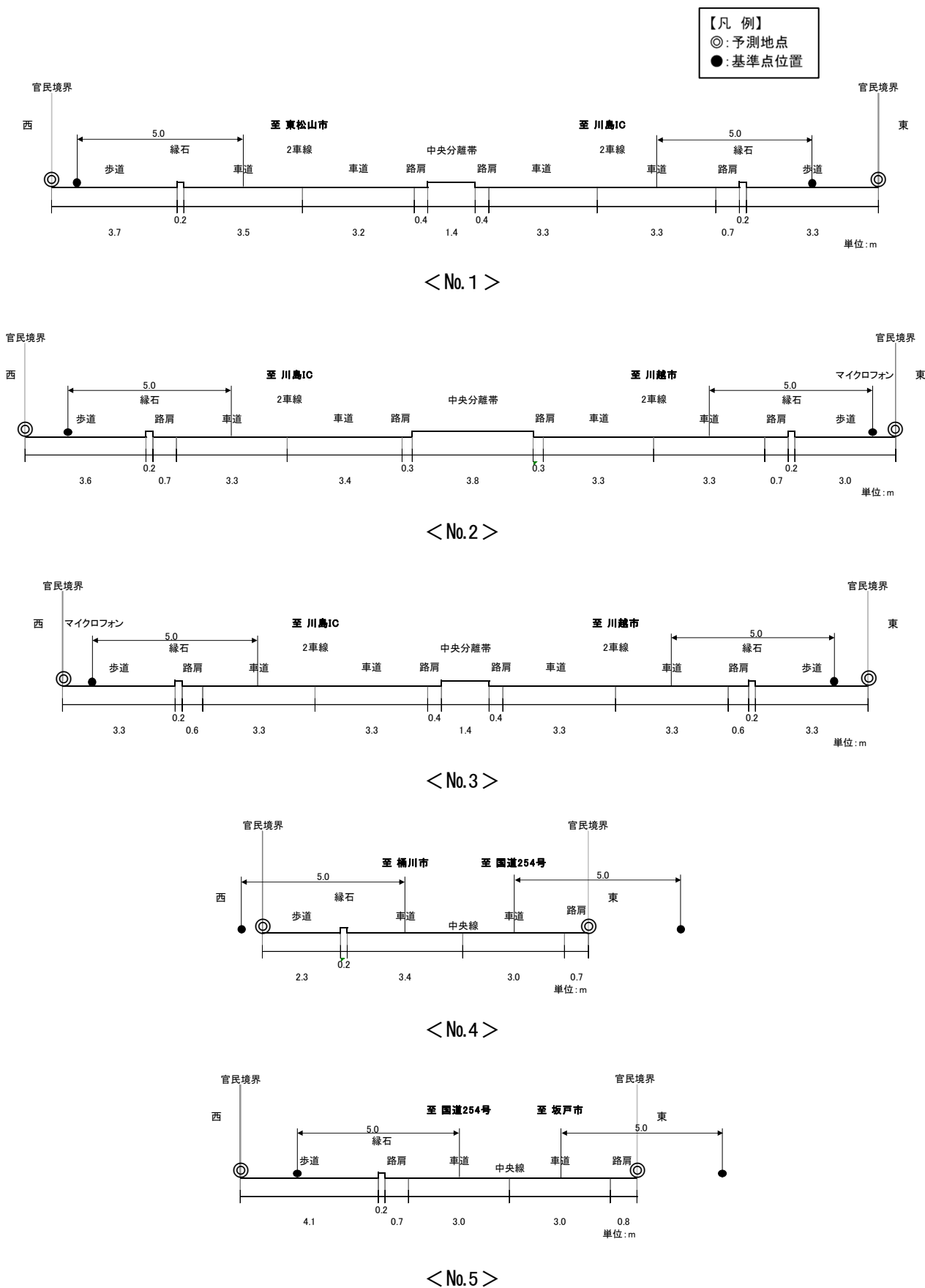
図 10.3.2-3 道路断面図
