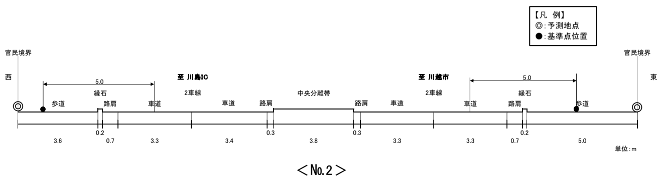
図 10.3.2-6 道路断面図
