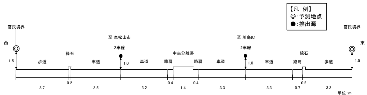
図 10.1.2-7(1) 道路断面図
