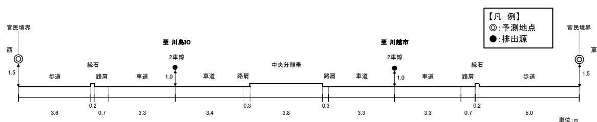
図 10.1.2-15 道路断面図
