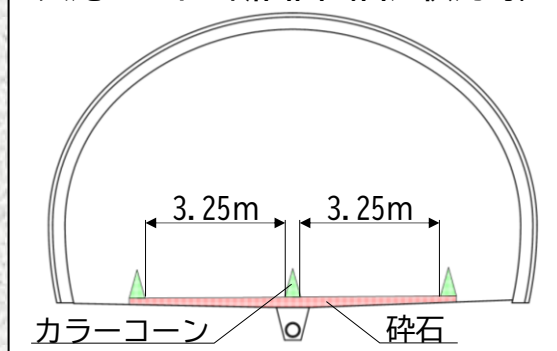
大滝トンネル断面図（暫定供用時）
