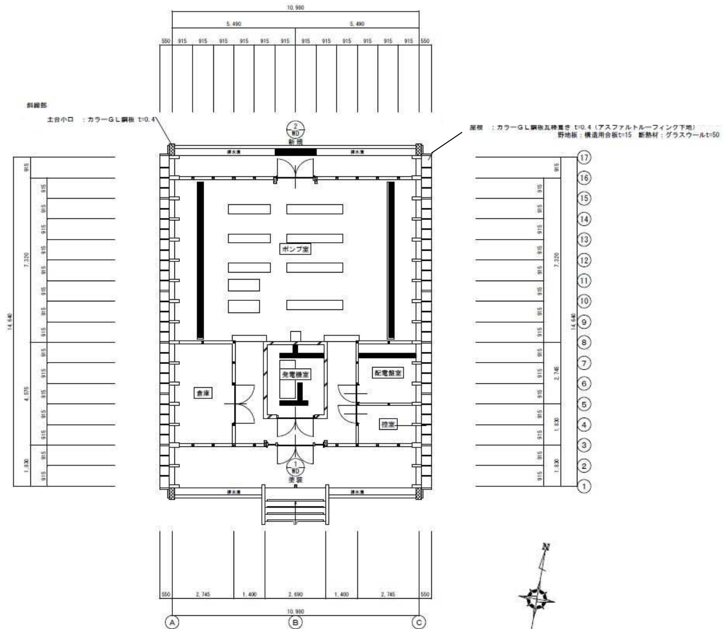
県民の森浄水場 平面図
