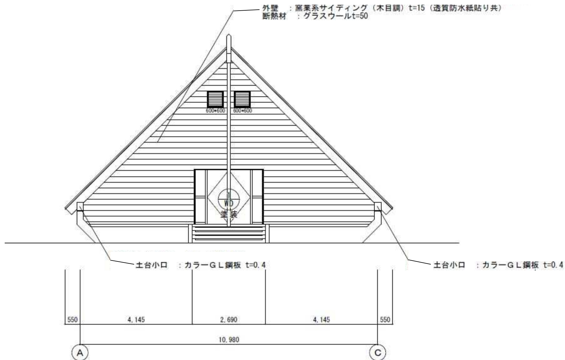
県民の森浄水場 立面図
