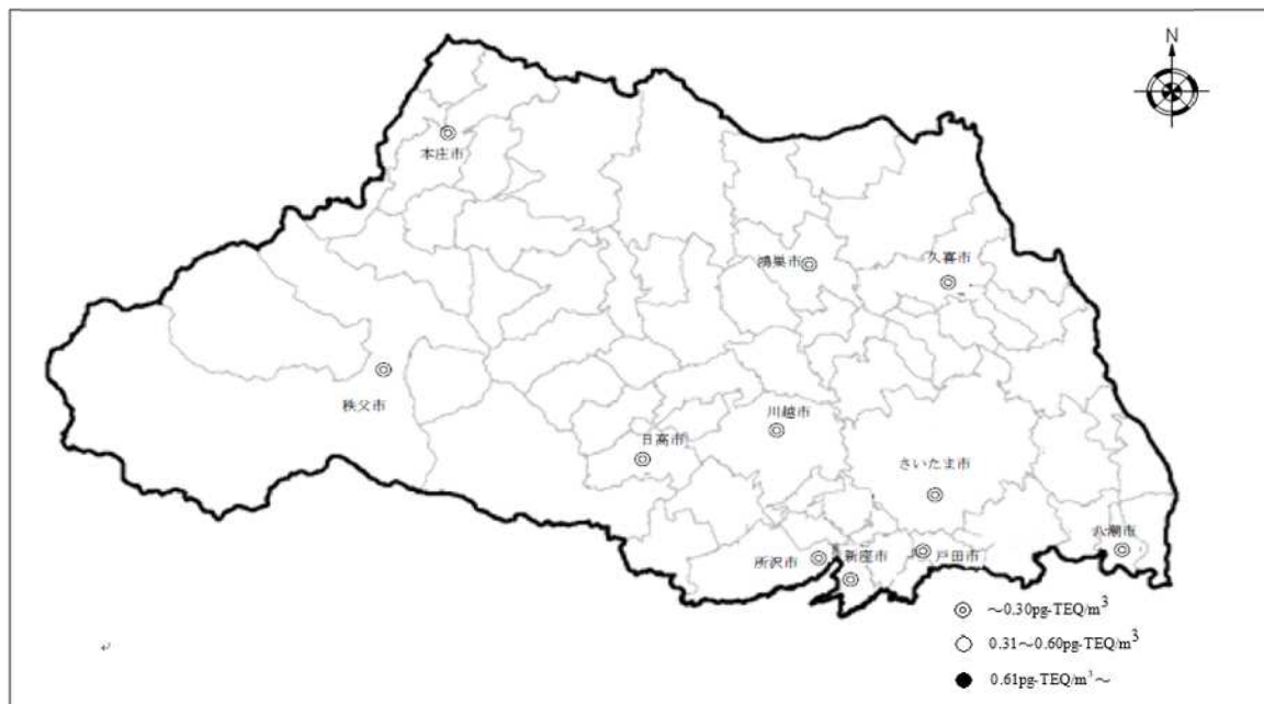
図Ⅲ－１ 令和６年度ダイオキシン類大気常時監視結果
