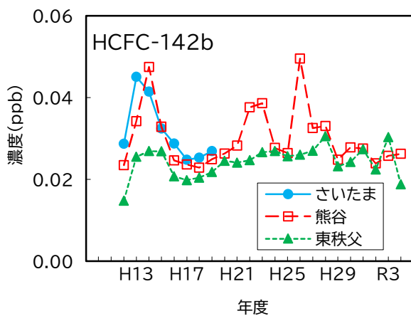
図16 HCFC-142b 濃度の経年変化
