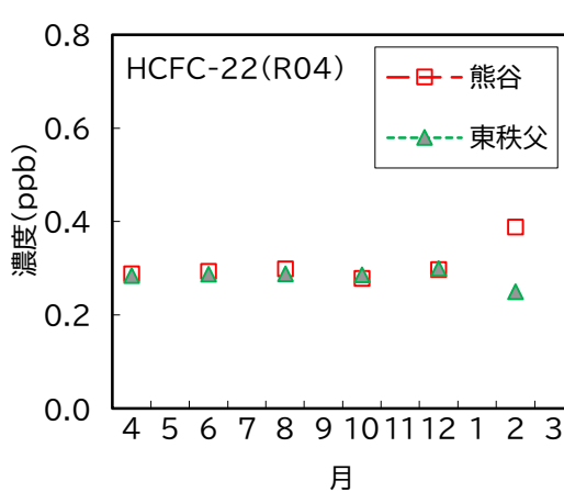
図13 HCFC-22濃度の経月変化
