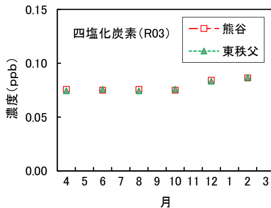
図11 四塩化炭素濃度の経月変化
