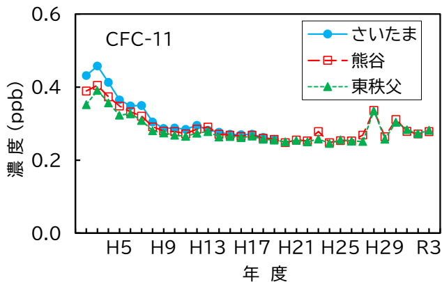
図2 CFC-11濃度の経年変化
