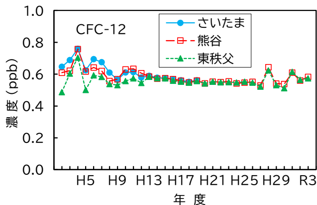
図4 CFC-12濃度の経年変化
