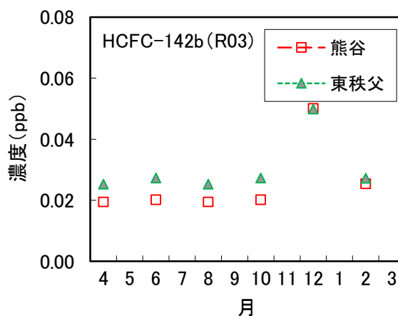
図17 HCFC-142b 濃度の経月変化
