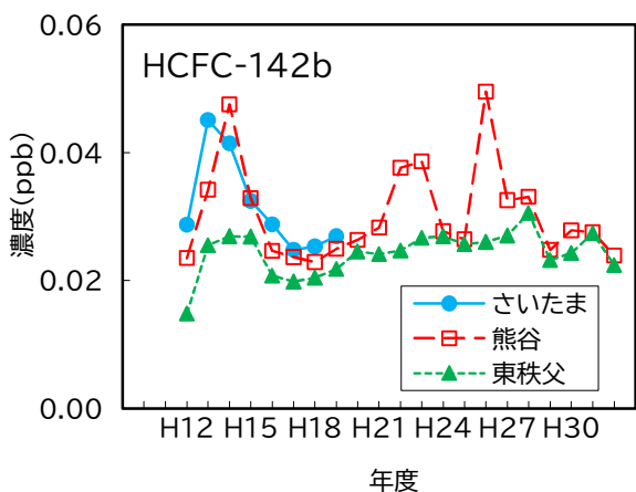
図16 HCFC-142b 濃度の経年変化
