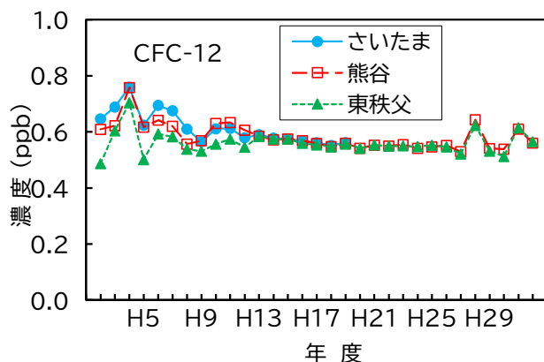
図4 CFC-12 濃度の経年変化
