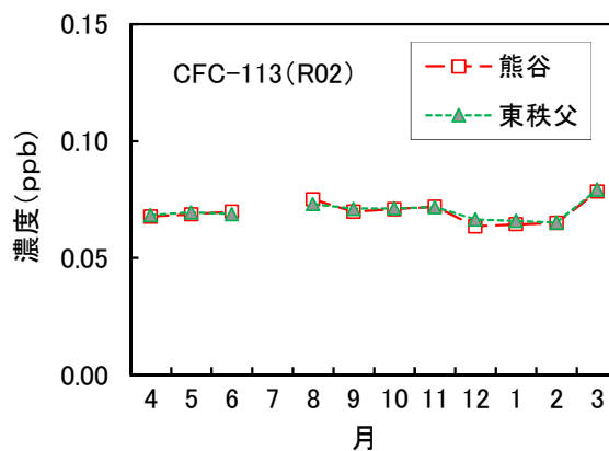
図7 CFC-113濃度の経月変化
