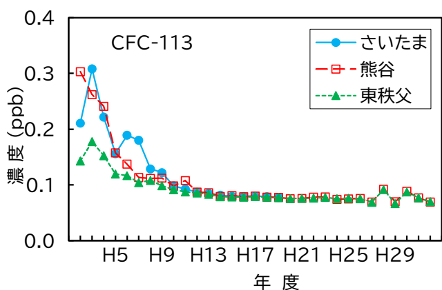
図6 CFC-113濃度の経年変化
