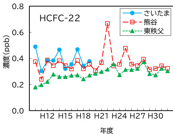
図12 HCFC-22濃度の経年変化
