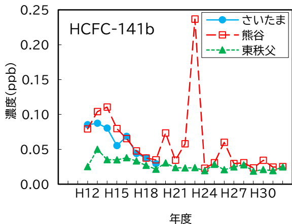
図14 HCFC-141b 濃度の経年変化
