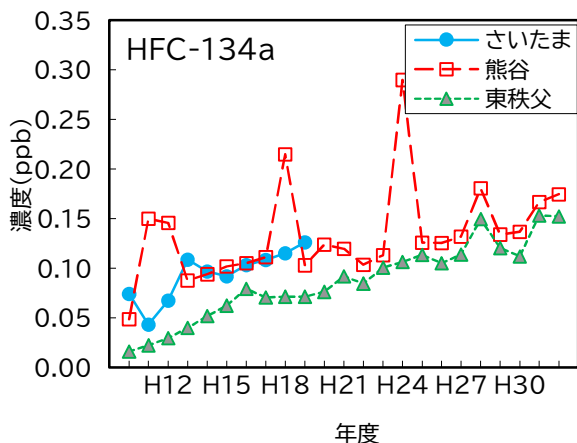
図18 HFC-134a 濃度の経年変化
