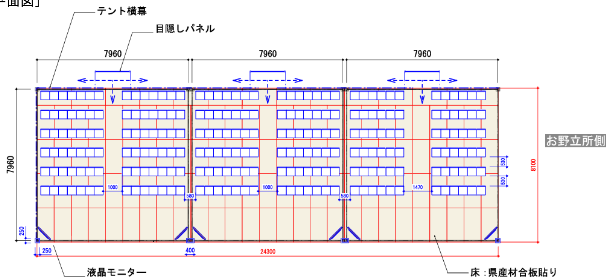
[平面図]
