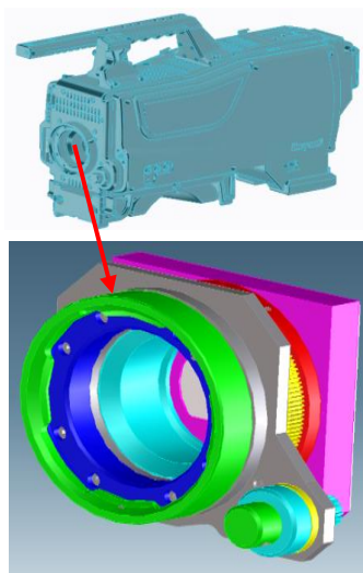
カメラ筐体と レンズマウント装置
