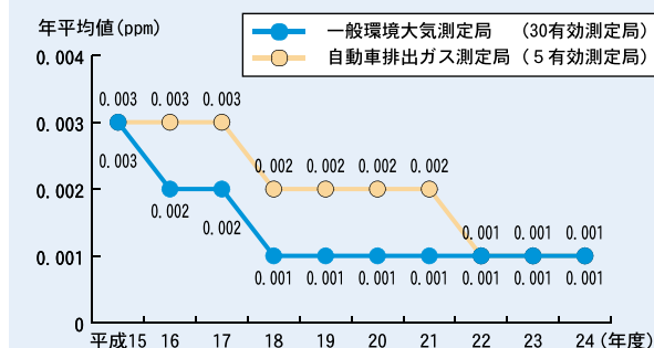
図1-1-4 二酸化硫黄の濃度の推移
