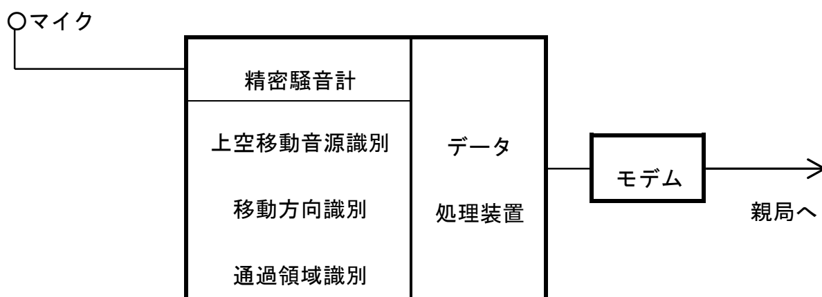
図－１－１ 測定システム概要（測定局）
