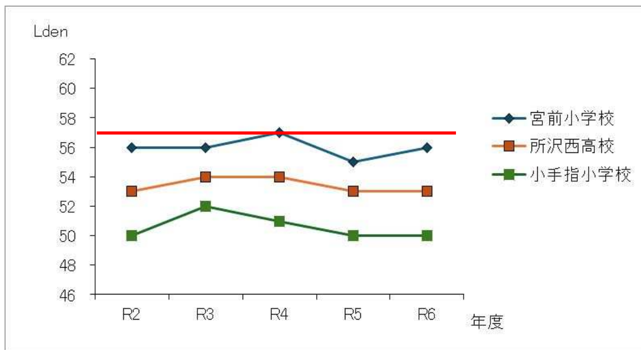
図-3 Ldenの推移(入間飛行場南側)
