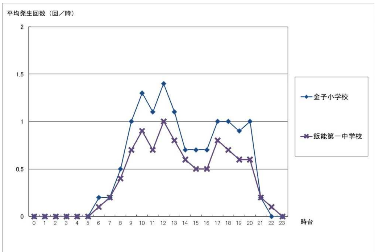
図－７ 時間帯別平均騒音発生回数（横田飛行場北側）
