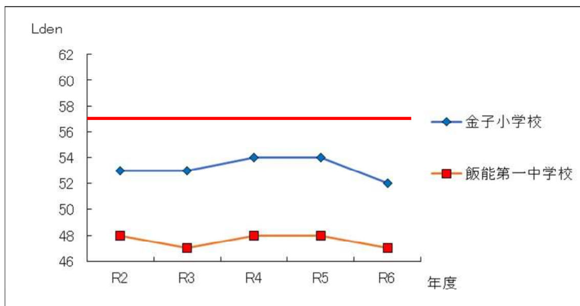
図-6 Ldenの推移(横田飛行場北側)
