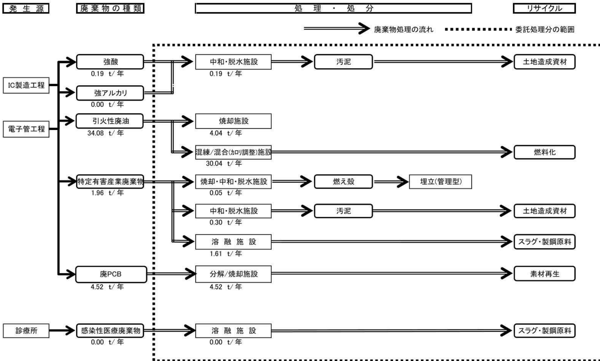
別紙2 特別管理産業廃棄物処理フロー図
