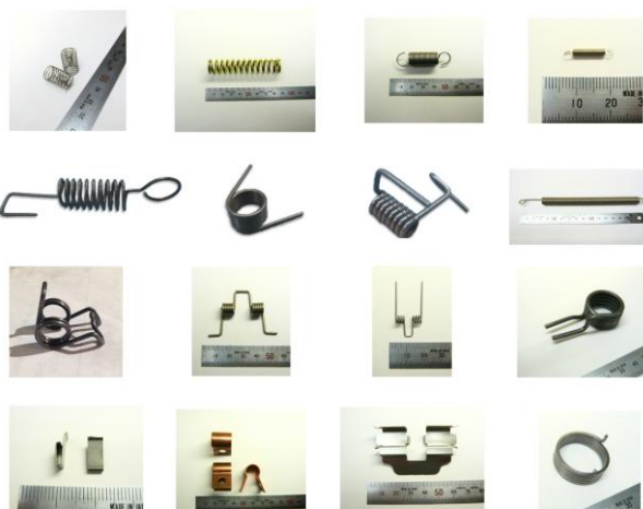
押しバネ/引きバネ/トーションバネ/ダブルトーションバネ
