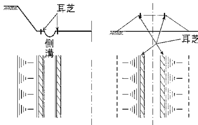
図 3-2-6 耳芝
