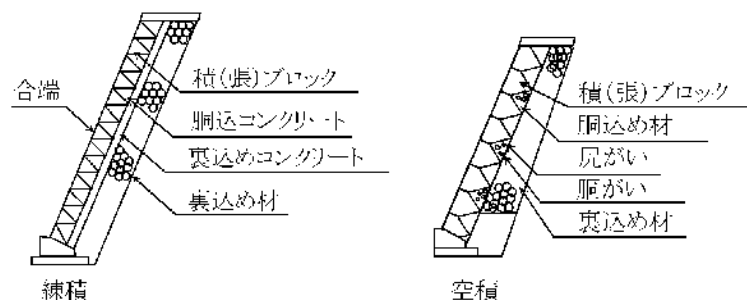
図3-2-5 コンクリートブロック工（標準図）
