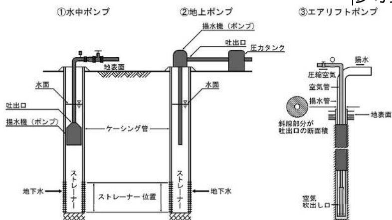
図－１ 揚水施設の主な形式
