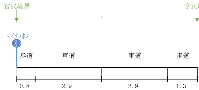
図 10.2-9(7) 道路構造図 (⑨)
