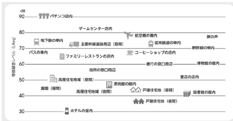
図 10.2-3 騒音の目安
