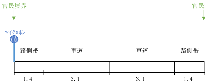
図 10.2-9(8) 道路構造図 (⑩)
