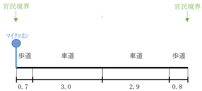
図 10.2-9(5) 道路構造図 (⑦)
