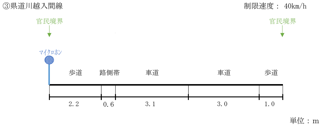
図 10.2-9(1) 道路構造図 (③)
