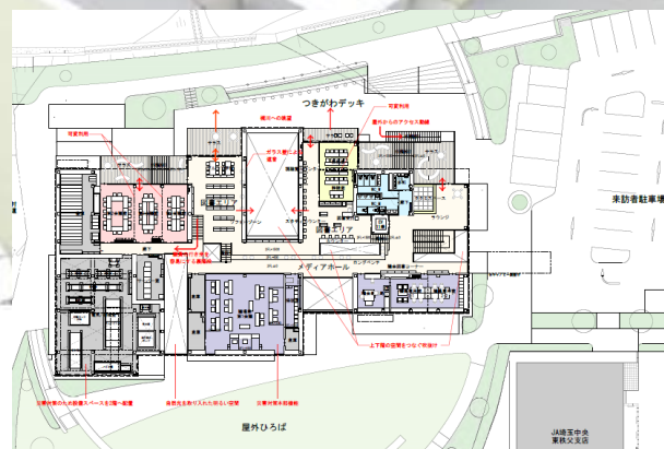
2階平面図
