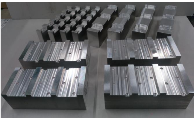
【量産を可能にしたオリジナル開発の治具各種】
