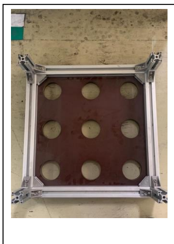
洗浄架台 アルミフレーム+板金ボルト締結
