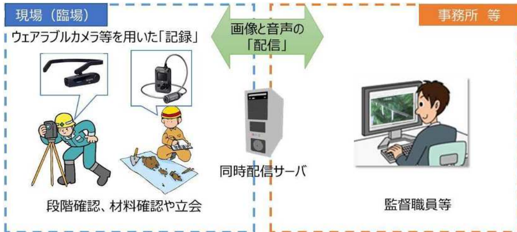
図 2-1 機器構成（例）
