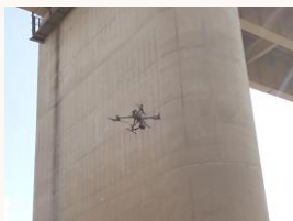
ドローンによる橋りょう点検
